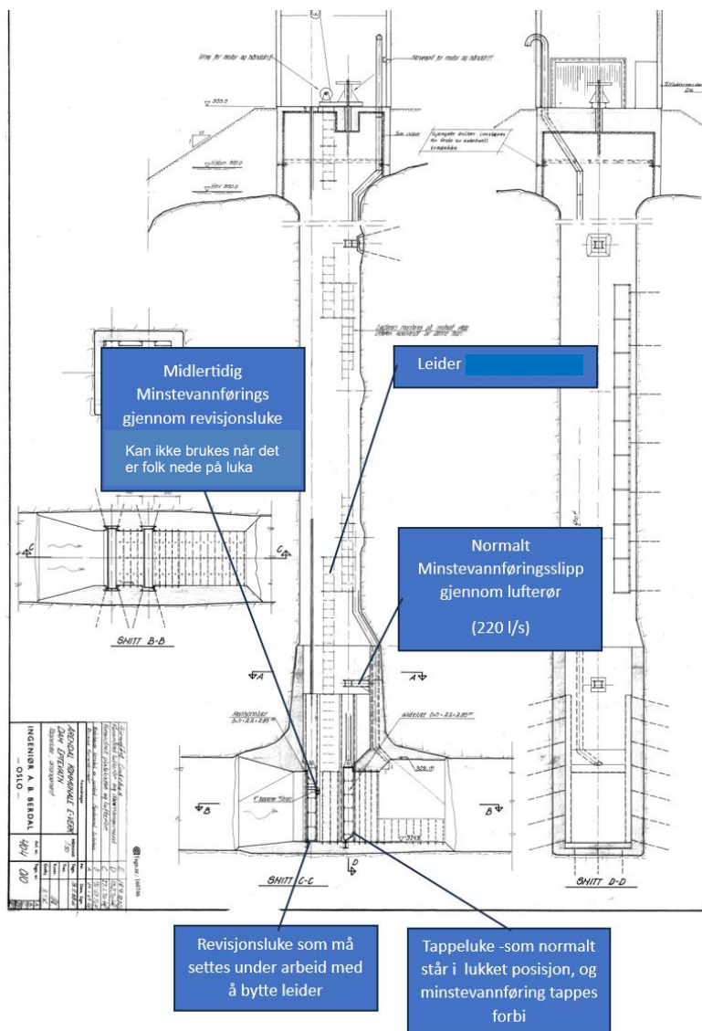
Figur 2 Illustrasjon minstevannføringslipp
