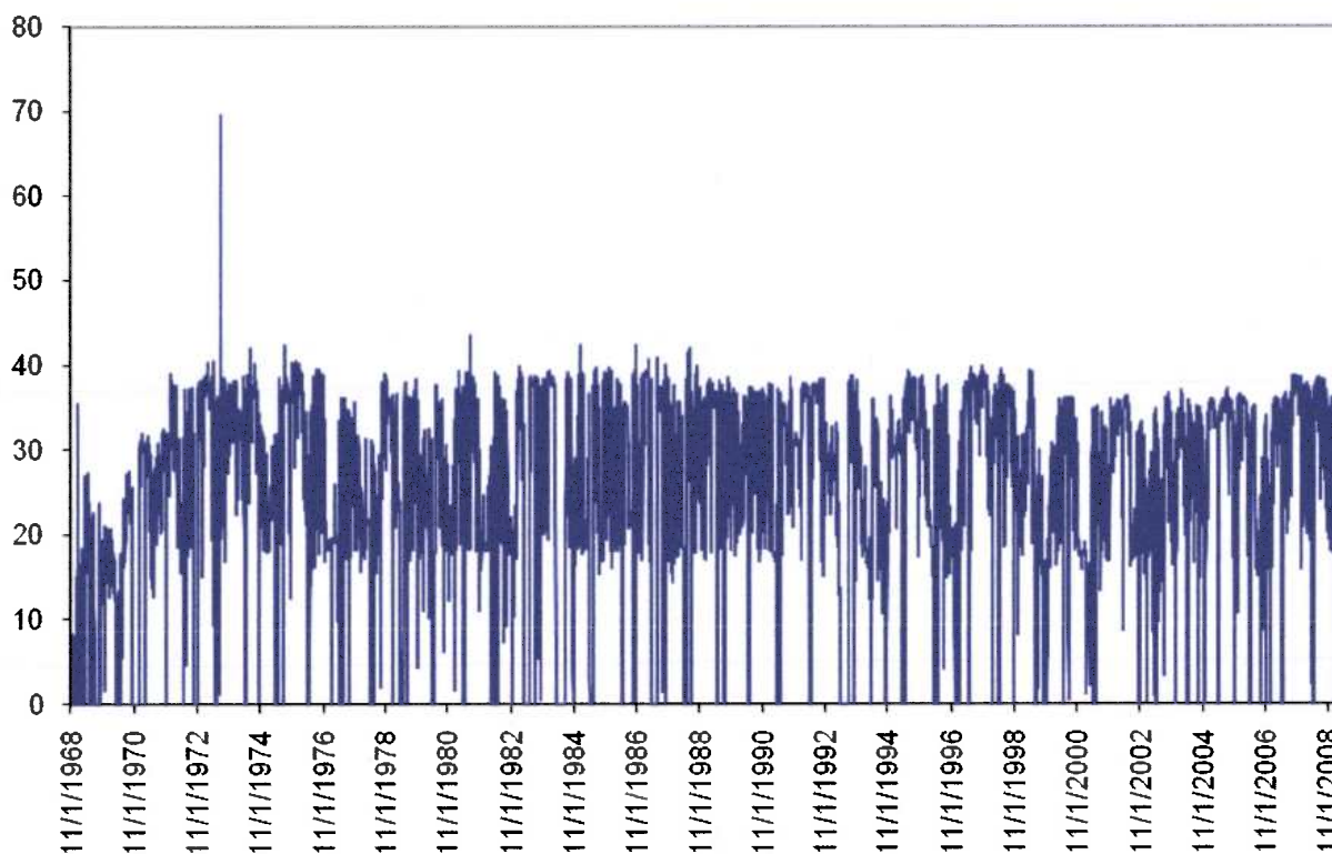
Figur 3Vannmengde m3/s produksjonsvann gjennom Trollheim kraftverk .
