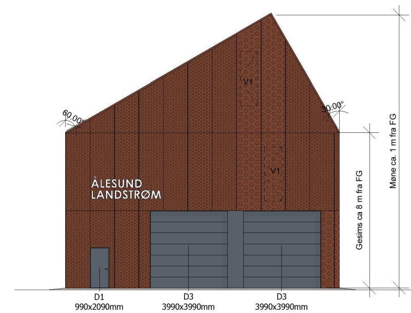
Fasade sør
