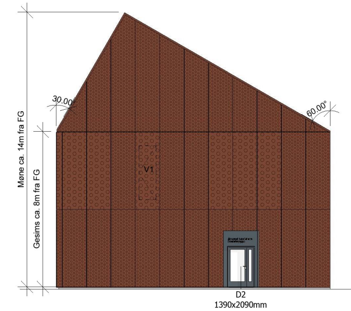
Fasade nord
