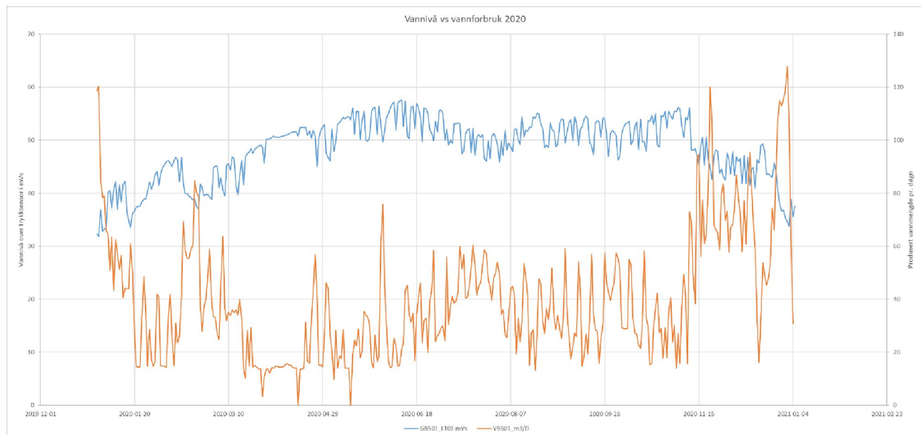
Figur 3: Vannivå i meter vannsøyle over sensor i brønn GB501 med blå graf og totalt vannforbruk i m 3 /døgn for begge brønnene GB501 og GB502 med oransje graf. Måleperiode 1.januar 2020 til 4.januar 2021.
