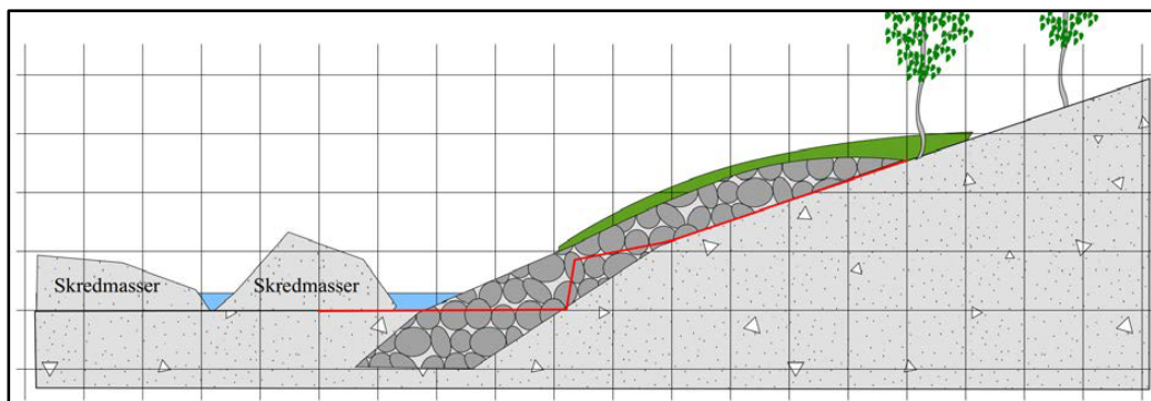
Figur 3: Prinsippskisse for utføring av sikring mot elv.
