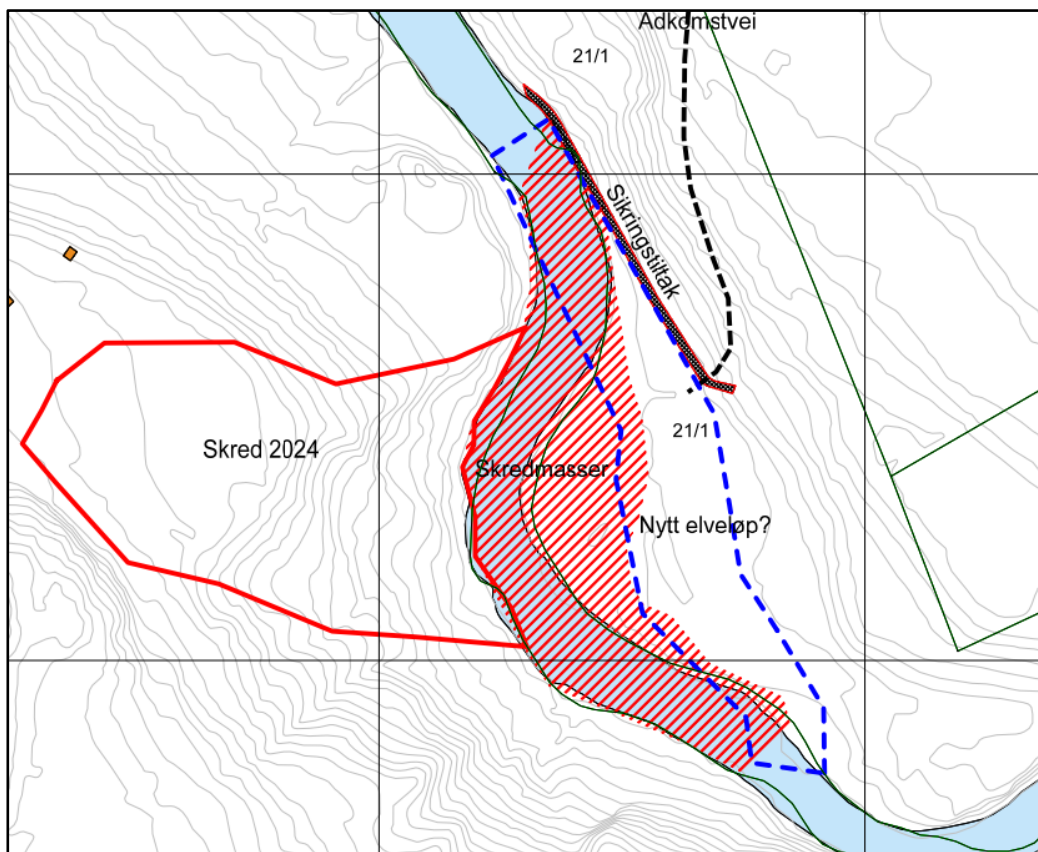
Figur 1: Oversiktskart over det planlagte tiltakets beliggenhet (svart og rød linje), adkomstvei (svart stiplet linje), skredområdet (innenfor rød heltrukket linje), skredmassene fra 2024 (skravert rødt område), og antatt nytt elveløp (innenfor blå stiplet linje). Nord er opp i figuren, og vannet renner nordover. Figur fra NVEs tiltaksplan datert 17.2.2025.
