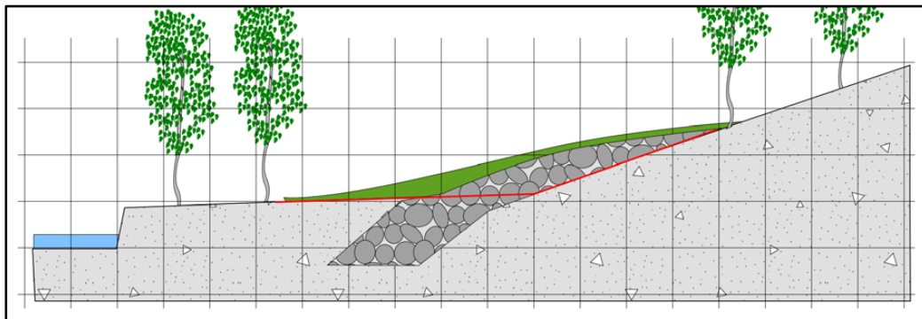
Figur 2: Prinsippskisse for utføring av sikring på land.
