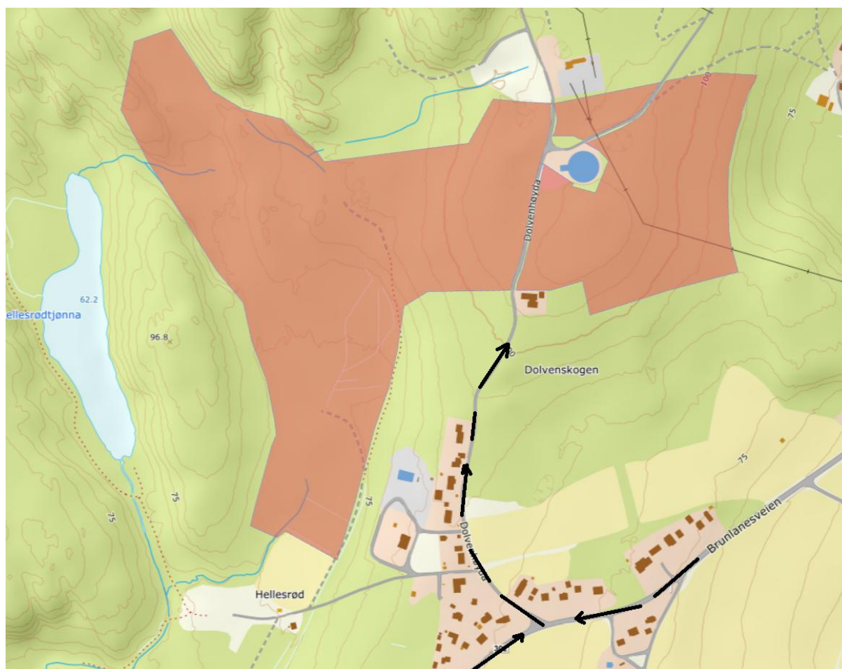
Figur 11 - Adkomst til solkraftverket
