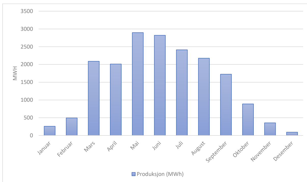
Figur 8 - Månedlig produksjon i Brunlanes solkraftverk
