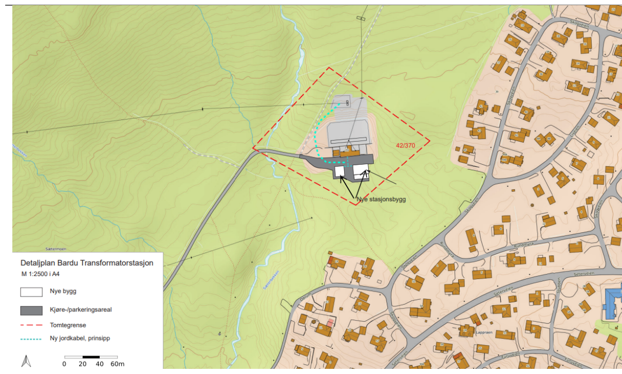
Figur 1: Oversiktskart av det omsøkte tiltaket.
