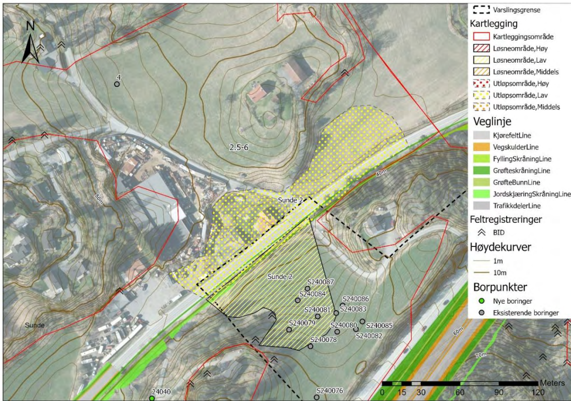
Figur 6-9: Opptegnet løsne- og utløpsområde for faresonen Sunde 2.
