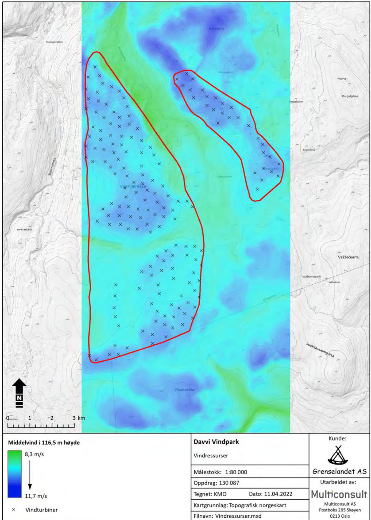
Govus 7-2. Plánaguovllu bieggakárta. Gaskamearrebiegga 116,5 m allodagas lea meroštallon leat 9,3 m/s, juoga mii lea hui buorre. Gáldu: Kjeller Vindteknikk.
