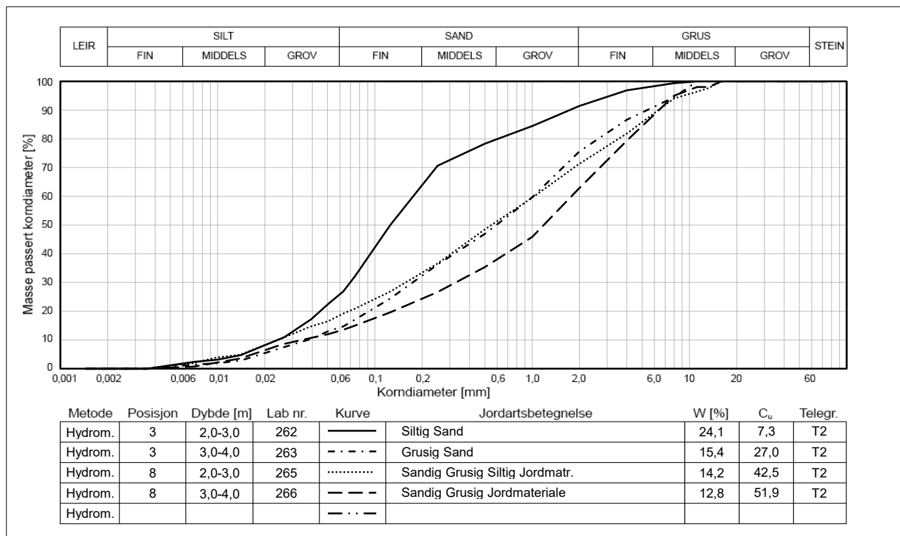
Figur 1 Korngraderingskurver i posisjon 3 og 8
