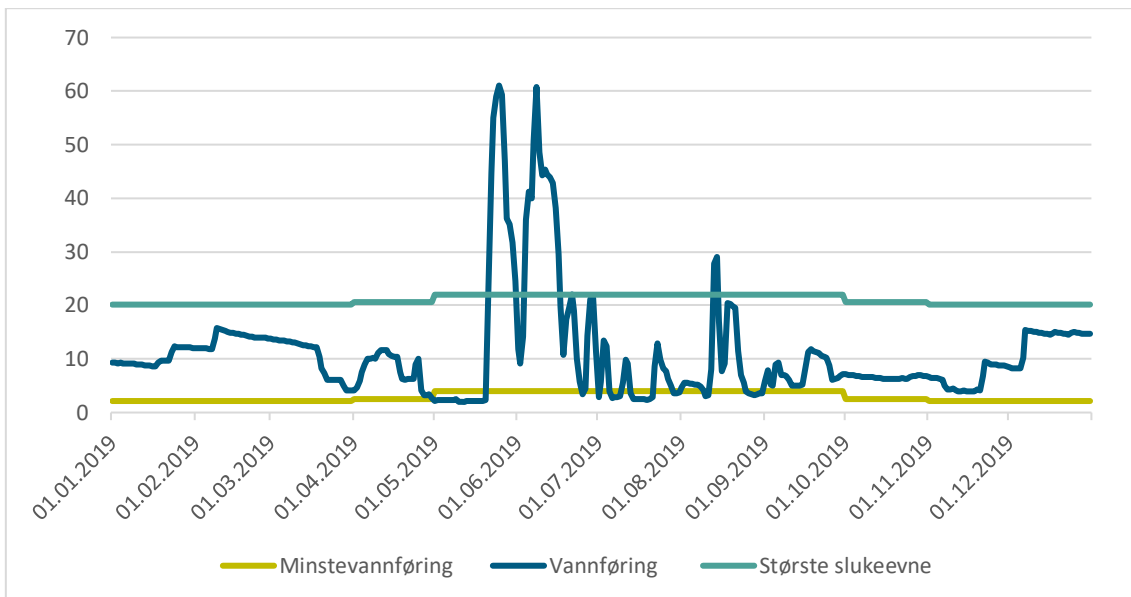
Figur 2-2. Oversikt over vannføring, minstevannføring samt største slukeevne over minstevannføring i 2019. Vannføringen er hentet fra Sildre [5]. Vannføring er gitt i m 3 /s.
