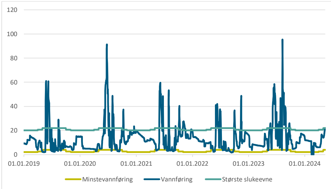
Figur 2-1. Oversikt over vannføring, minstevannføring samt største slukeevne over minstevannføring i perioden 01.01.2019 til 13.05.2024. Vannføringen er hentet fra Sildre [5]. Vannføring er gitt i m 3 /s.
