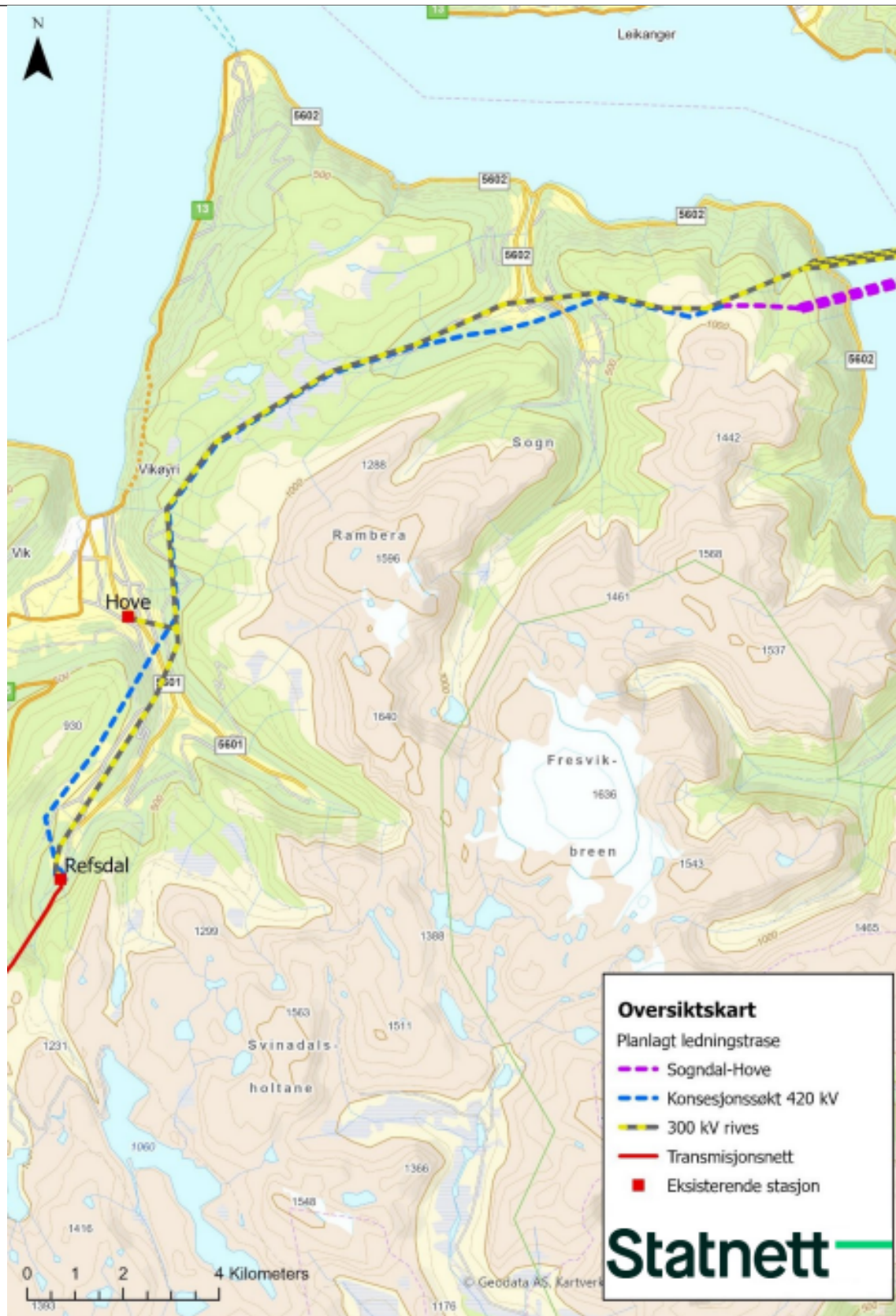
Figur 1: Oversiktskart ny 420 kV kraftledning Ramnaberg–Vik. Kjelde: Statnett sin konsesjonsøknad.
