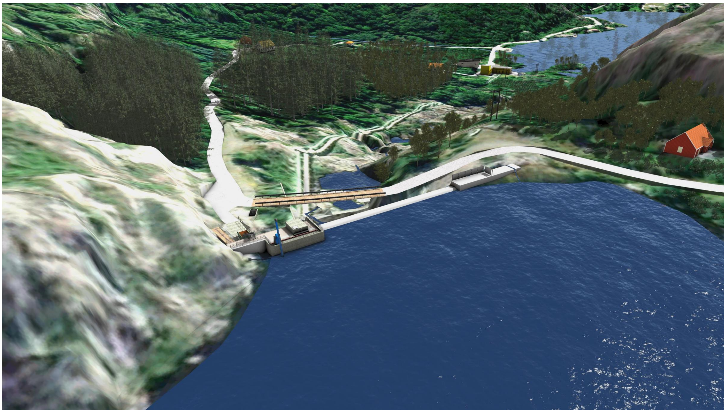
Illustrasjon som syner dam og inntaksområdet frå oppstraums side etter utbygging. Kraftstasjonsområdet er synleg øvst i bilete.
