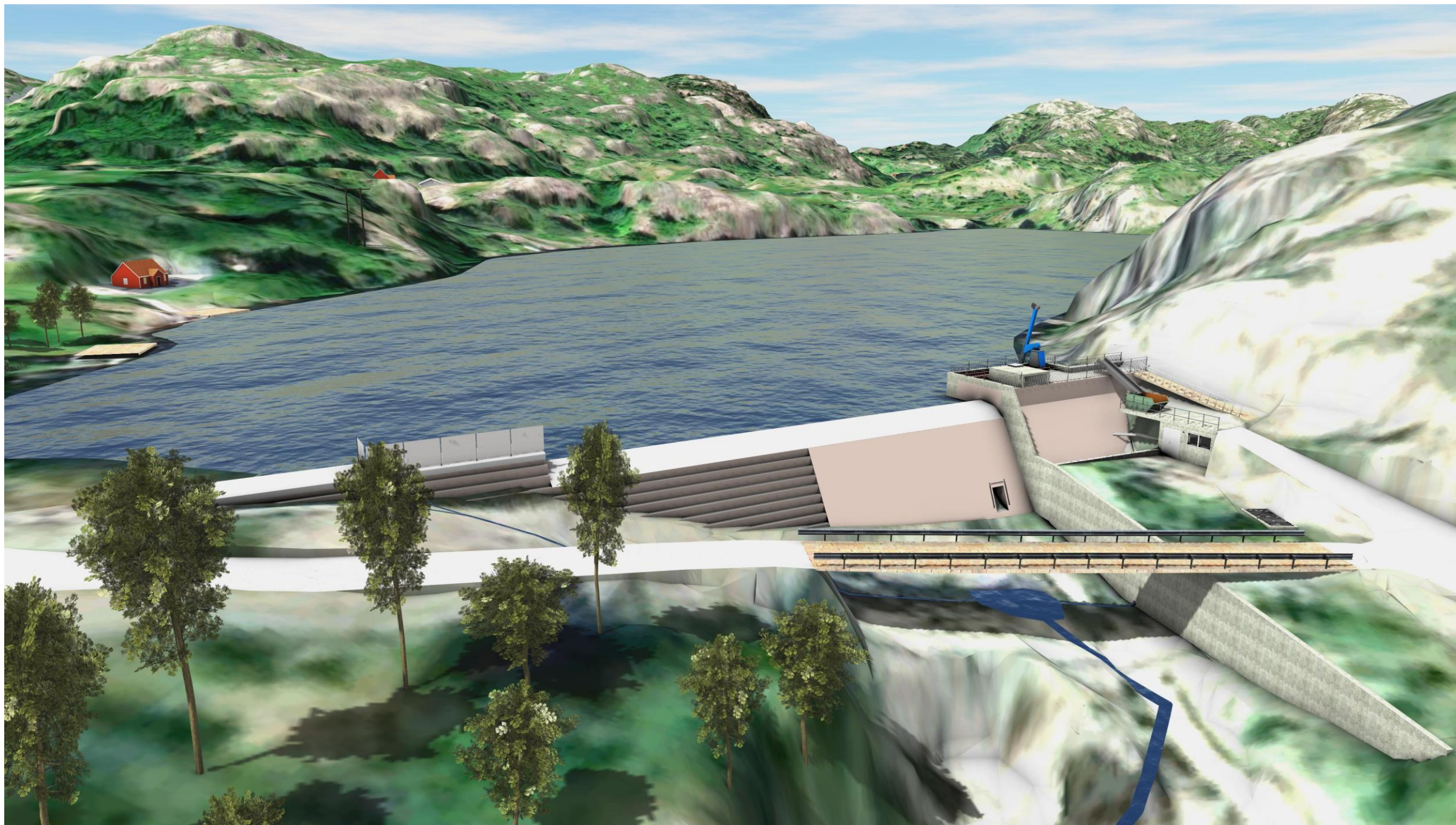
Illustrasjon som syner dam og inntaksområdet frå nedstraums side etter utbygging.
