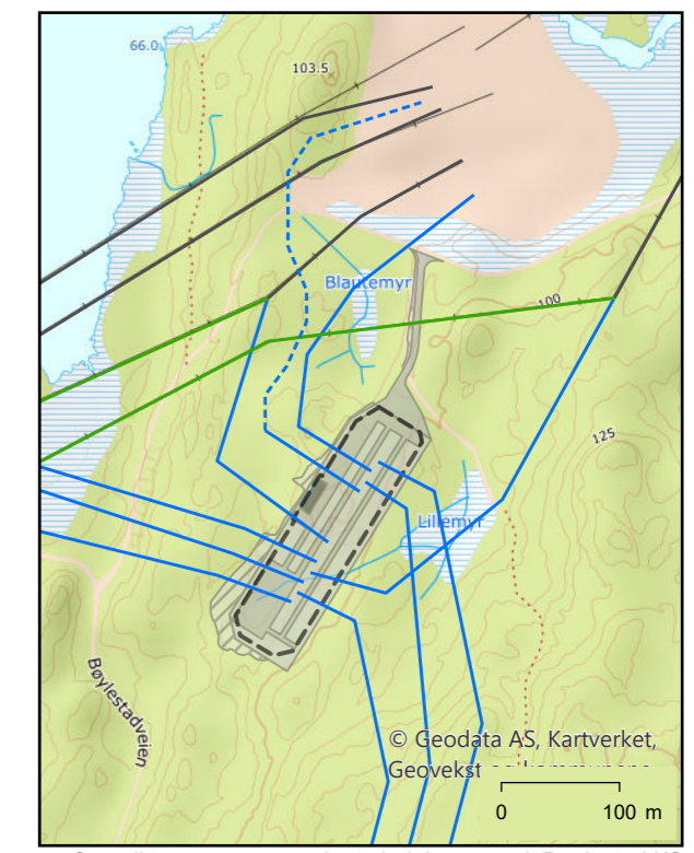
Oversikt over nye og omlagte ledninger rundt Bøylestad KS
