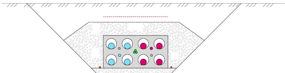
Figur 2. Snitt kabelkanal, Såheim-Vestfjorddalen.
