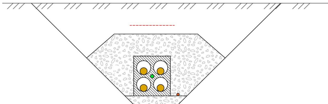
Figur 3. Snitt kabelkanal, Vestfjorddalen-Rjukan næringspark (T5).
