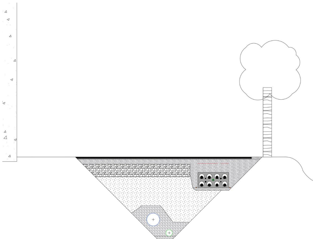
Figur 1. Snitt, Såheim-Vestfjorddalen, inkl. vannledning, kabelkanal, bjørketrær og vernet stolpe.
