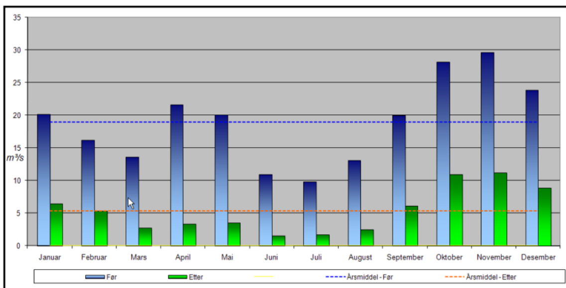
Figur 3-1 Månedsmiddel vannføringer (1971-2009) i m³/s før og etter tiltak.
