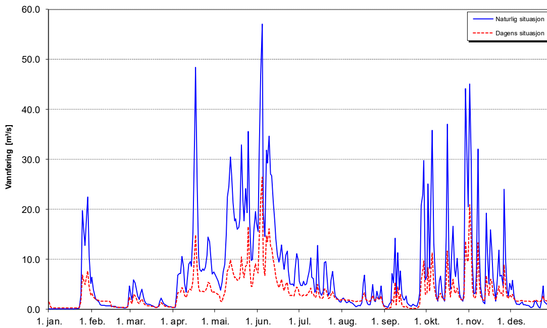
Tverråga i referansepunkt for øvre del av anadrom strekning - vått år - 2011
