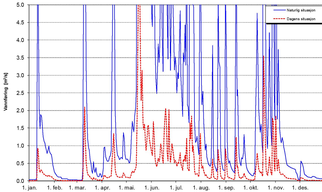
Tverråga like oppstrøms Rauvatnet - tørt år - 2010
