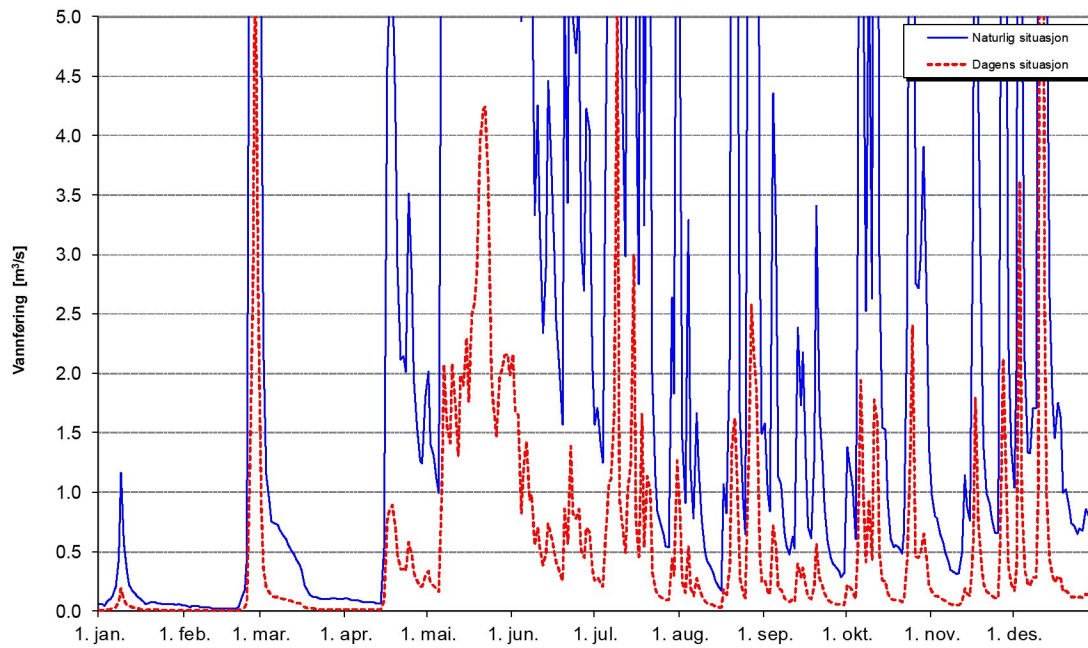
Tverråga like oppstrøms Rauvatnet - middels år - 2013
