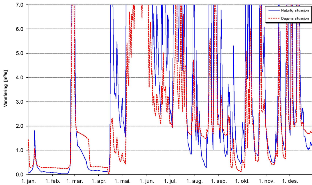
Tverråga i referansepunkt for øvre del av anadrom strekning - middels år - 2013
