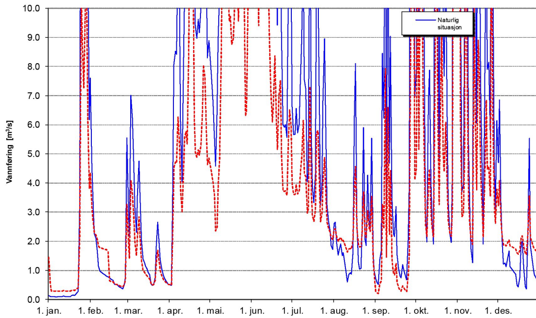
Tverråga like oppstrøms utløp i Rana - vått år - 2011
