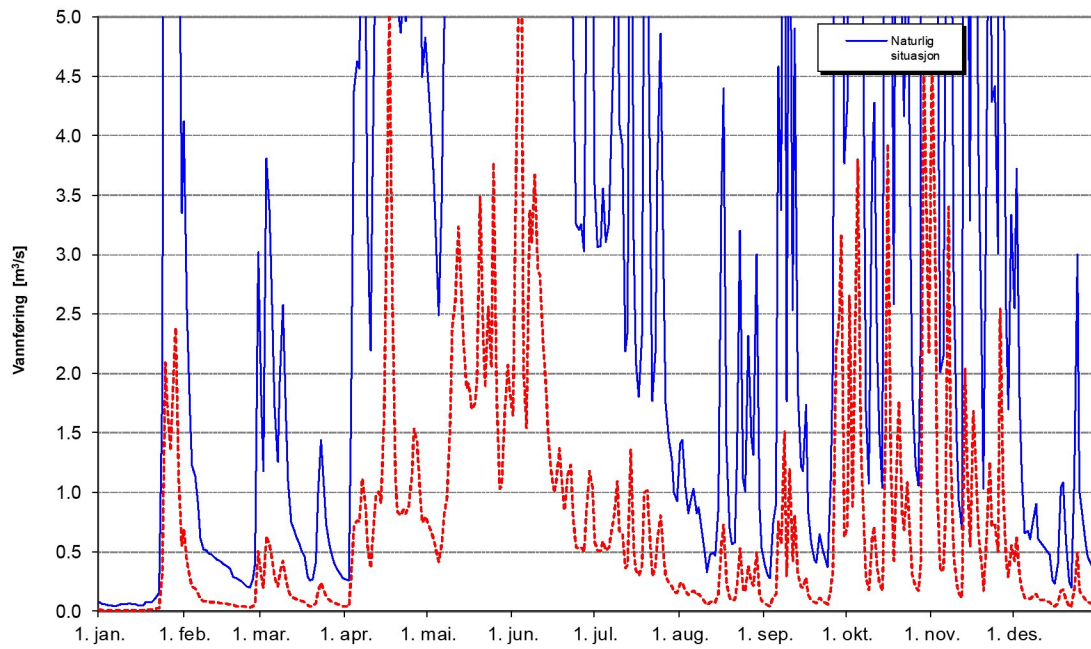
Tverråga like oppstrøms Rauvatnet - vått år - 2011
