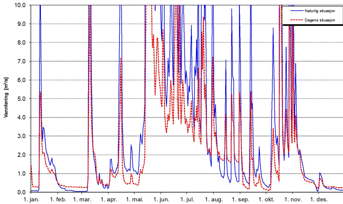
Tverråga like oppstrøms utløp i Rana - tørt år - 2010
