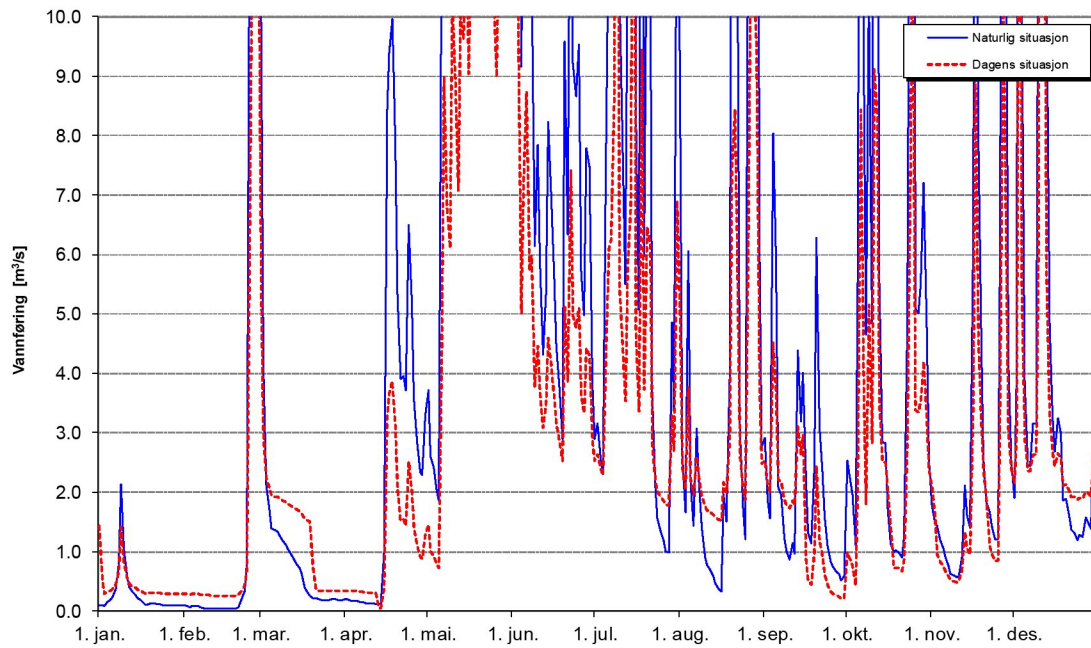
Tverråga like oppstrøms utløp i Rana - middels år - 2013
