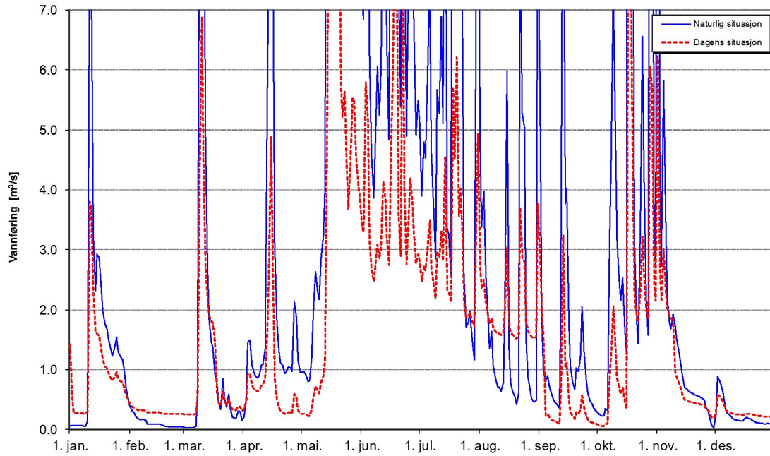
Tverråga i referansepunkt for øvre del av anadrom strekning - tørt år - 2010
