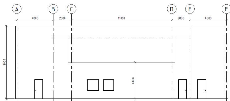
Fasade Sør 1 : 100
