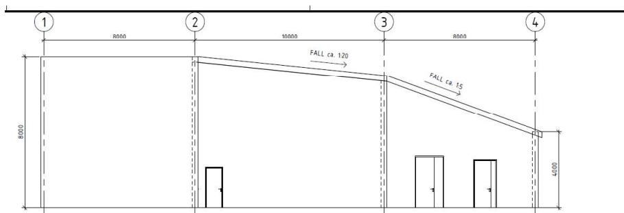
Fasade Vest 1 : 100
