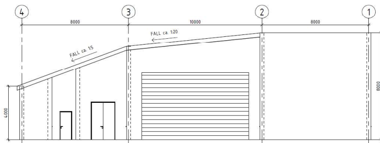
Fasade Øst 1 : 100
