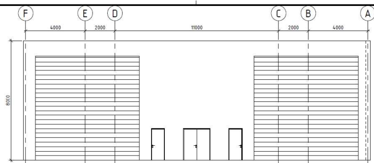
Fasade Nord 1 : 100
