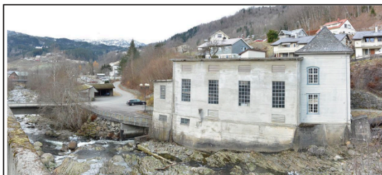
Figur 2-10: Etter utviding på 50-talet står den øvre delen igjen som den einaste originale, med trekledning. Ny bygningsmasse har eit meir funksjonalistisk preg og er utført i betong. Hovuddelen er vorten både breiare og lengre, slik at kraftstasjonen har sprang i sideretning og beslaglegg større del av elveleiet. Elveleiet har lite kantvegetasjon.
