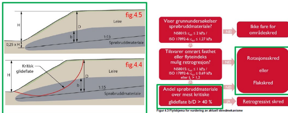
Figur 4. Utklipp fra NVE's veileder figur 4.4 og 4.5, samt flytskjema for vurdering av skredtype.
