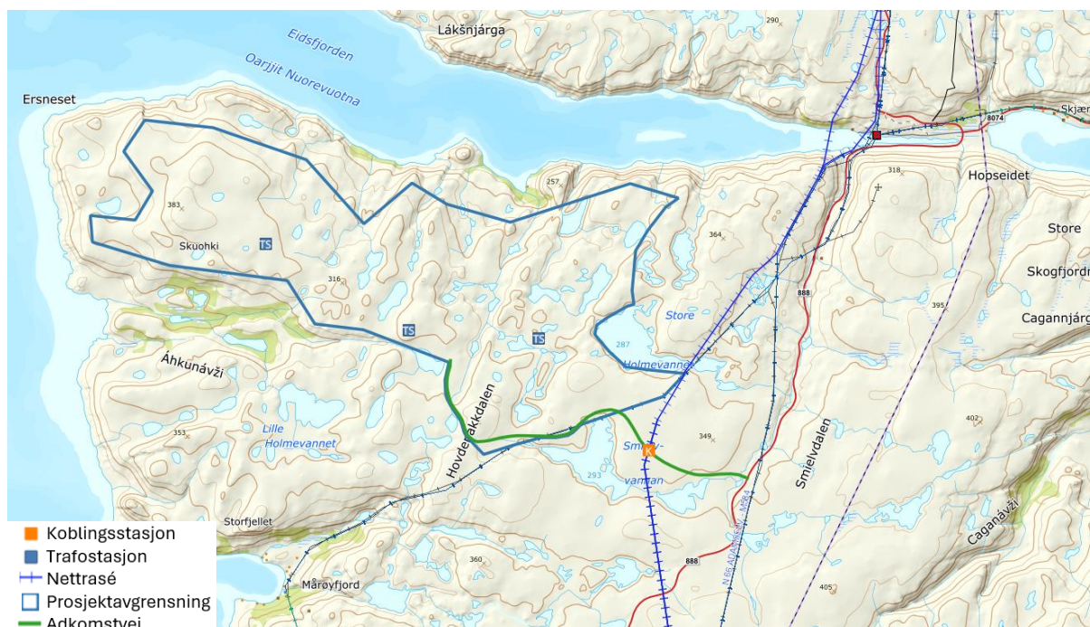
Figur 8. Foreslått stasjonsløsning for Laksefjorden vindkraftverk, med foreløpige trafoplasseringer.
