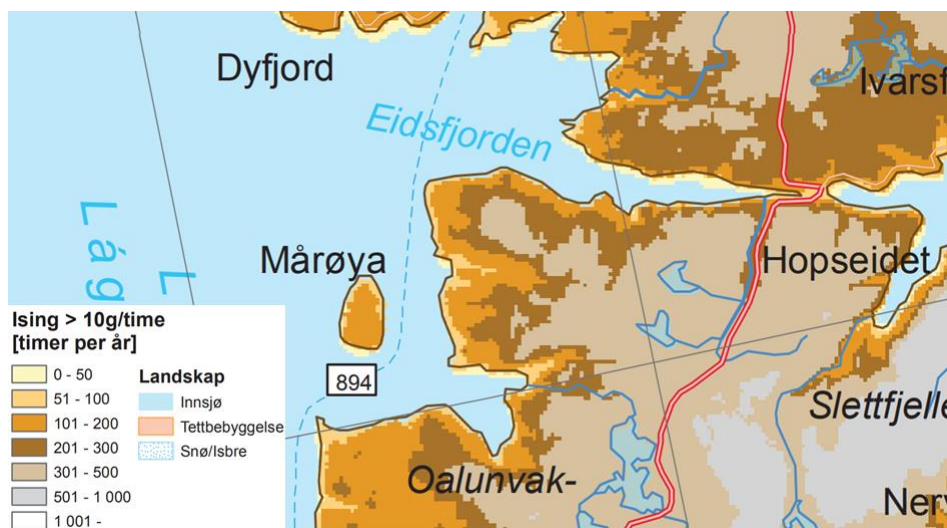
Figur 10. Ising > 10 g/time for området rundt Laksefjorden (Kjeller Vindteknikk, 2009).
