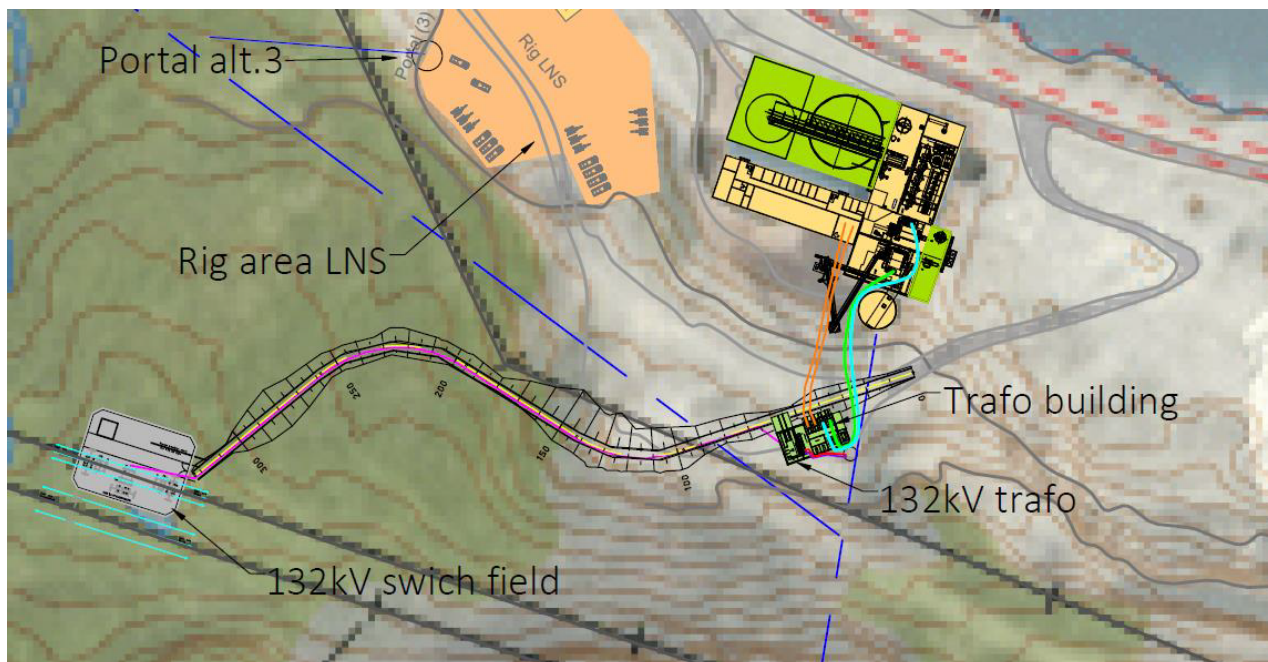
Figur 2: Illustrasjon over plassering av Lucernas omsøkte koblingsstasjon og ny Øyen transformatorstasjon. Kilde: søknaden.
