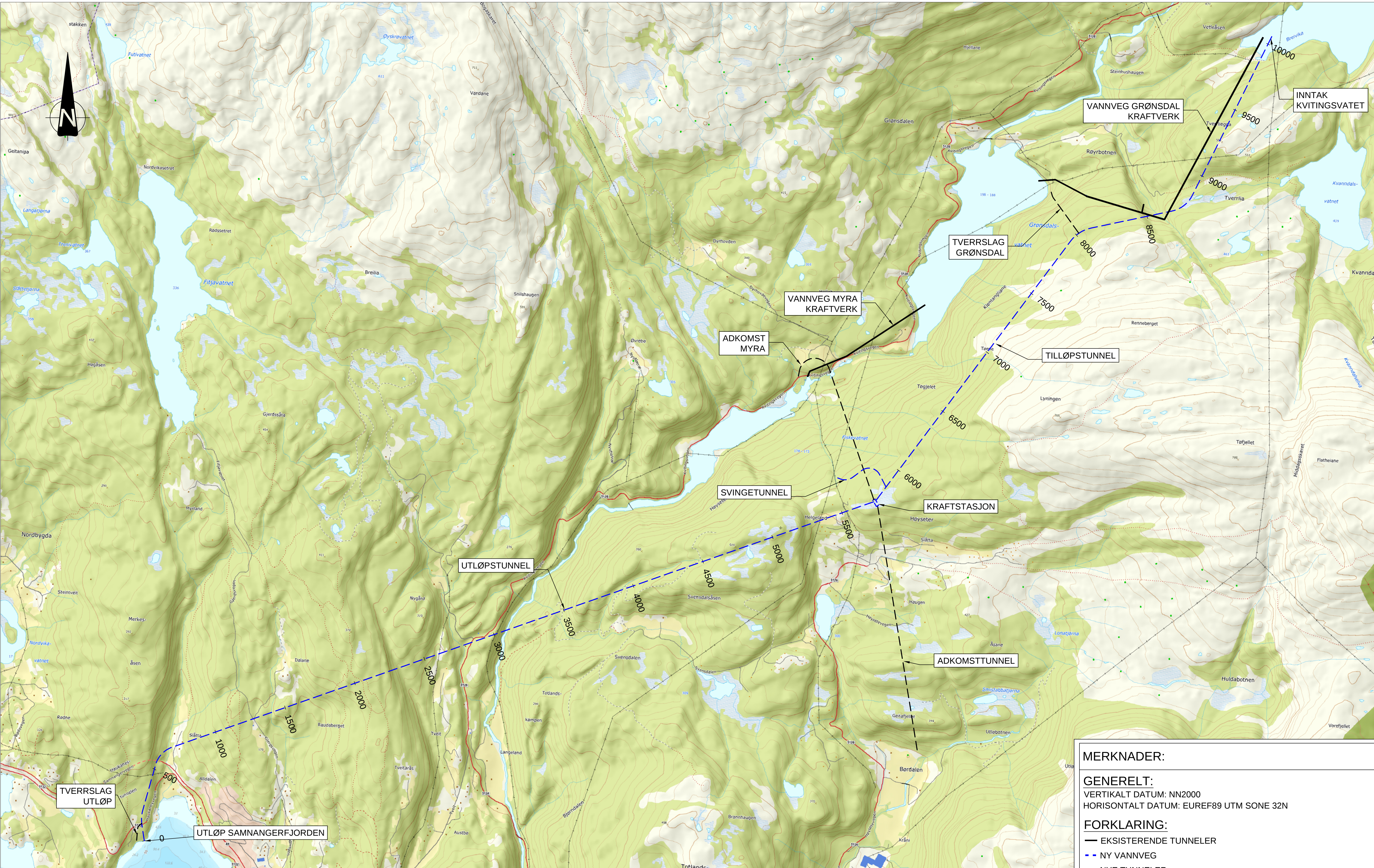
BØRDALEN KRAFTVERK - PLAN 1:12 000
