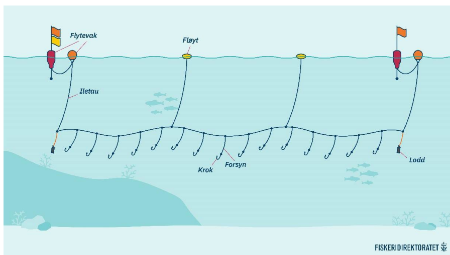
Figur 18 Fløyline og dets komponenter (Fiskeridirektoratet, 2022).
