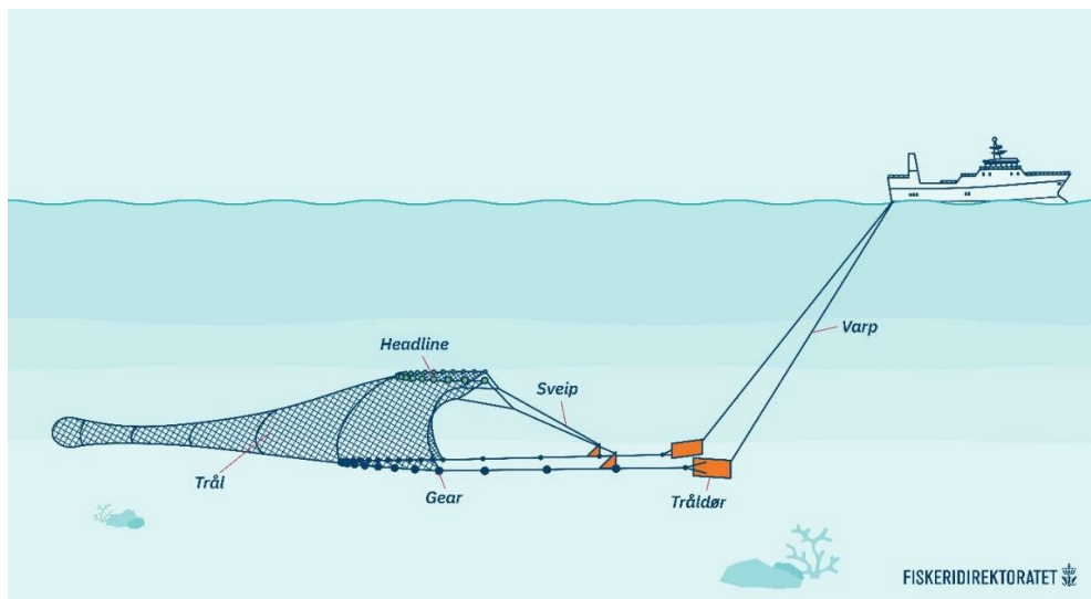
Figur 11 Bunntrål med komponenter (Fiskeridirektoratet, 2022).
