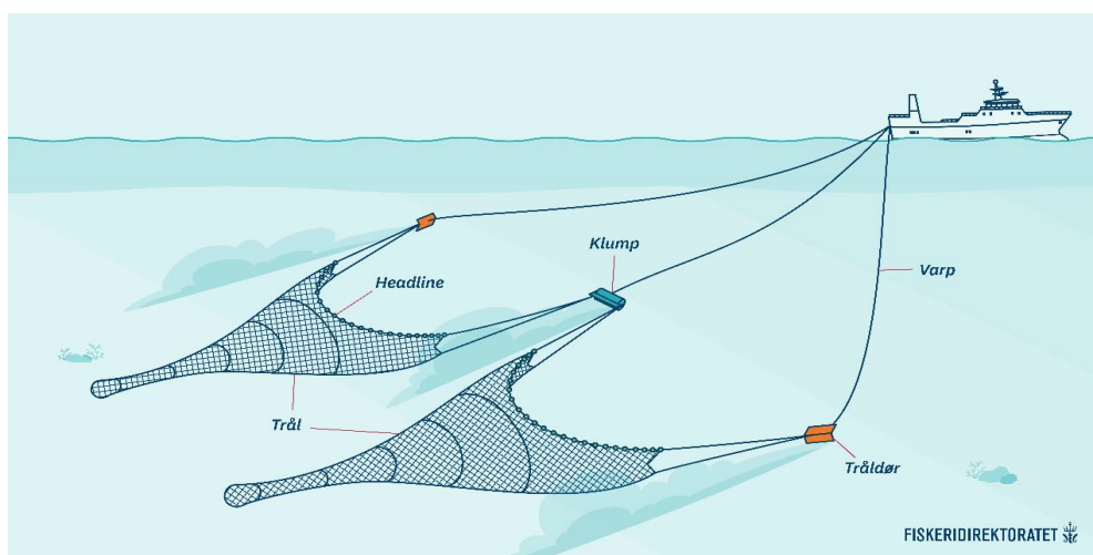
Figur 12 Dobbelt bunntrål og viktige komponenter (Fiskeridirektoratet, 2022).
