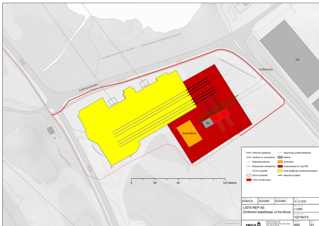
Figur 1: Kabeltrasé ut av transformatorstasjonen ved Alcoa. Ny trasé er vist med heltrukket rød strek, eksisterende er vist med stiplet strek.
