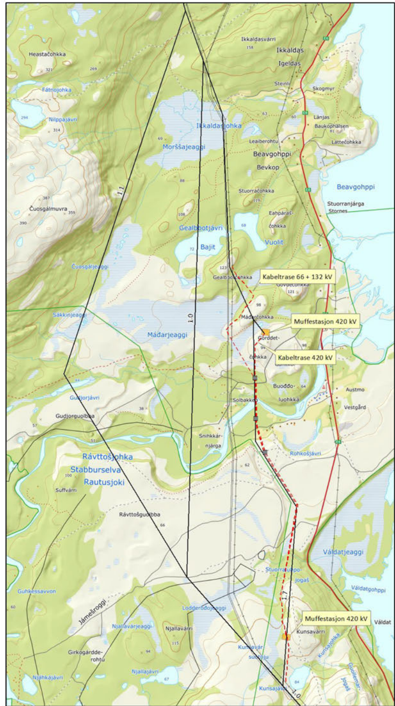
Figur 2-12. Alternative løsninger for kryssing av Stabbursdalen. Rød, stiplet linje angir mulige jordkabeltraseer.
