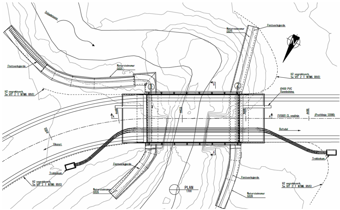
Figur 1: Planteing ny Fosse bru.
