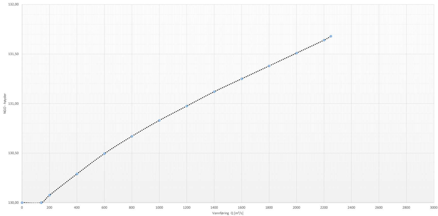
Vannføringskurve for Funnefoss overvann - Kurve 5 korrigert for avvik mellom v.m lensefeste og v.m inntak etter observasjoner 1991 - 1995
