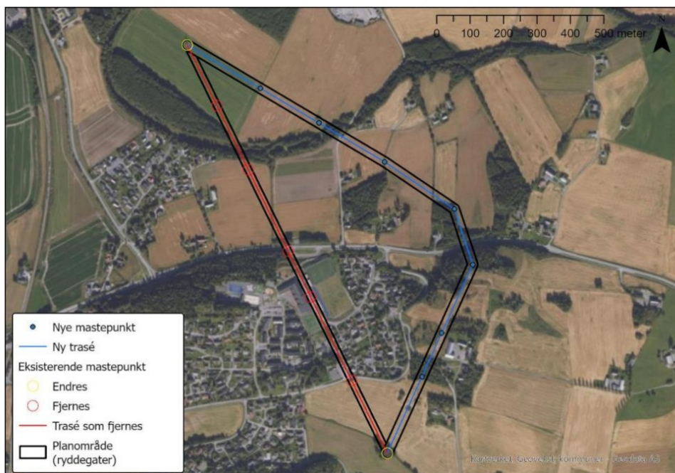
Figur 1: Ny kraftledningstrasé markert i blått. Eksisterende ledning som skal rives markert i rødt.
