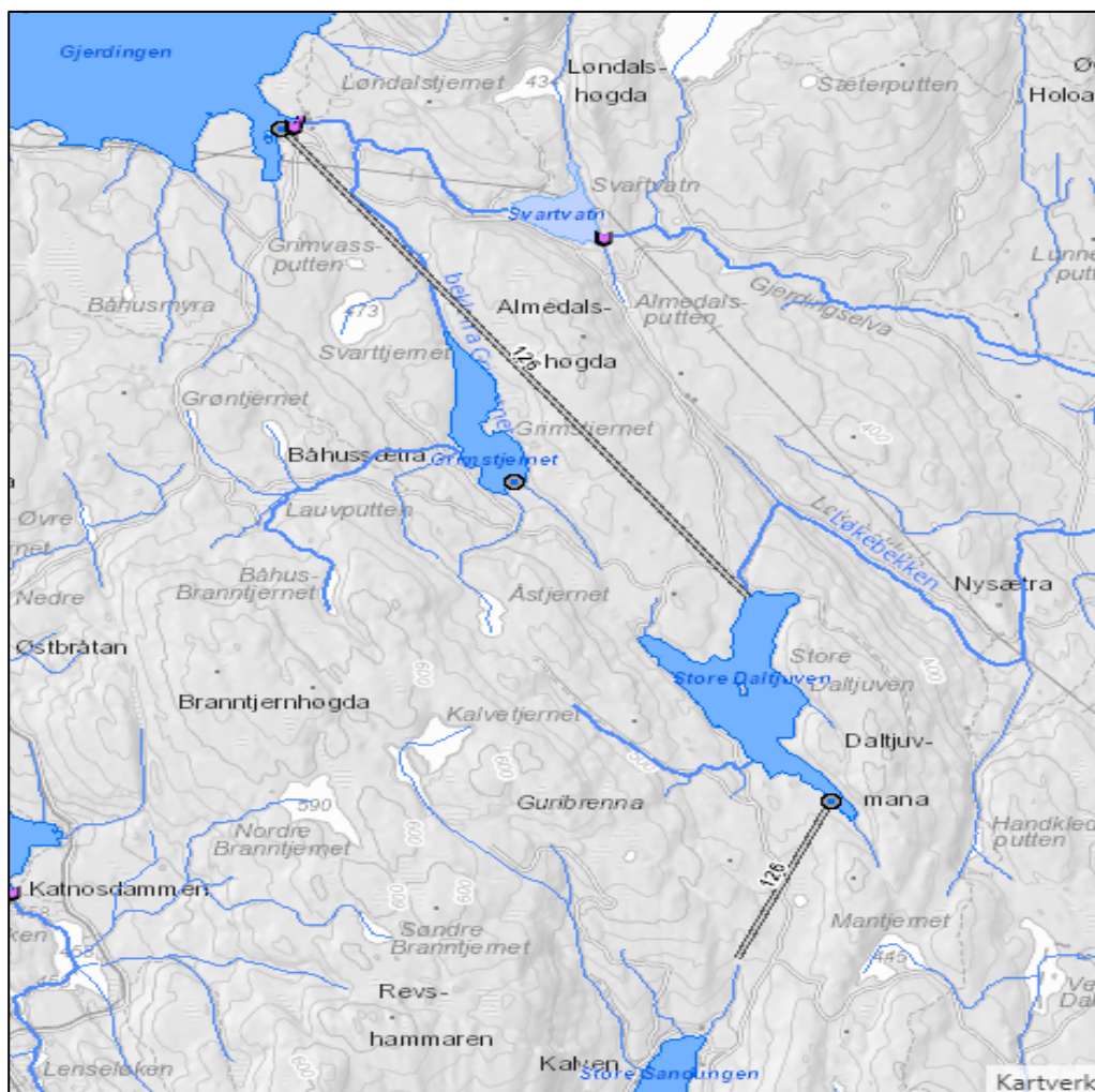
Figur 1. Overføringstunnelene Gjerdingen-Store Daltjuven og Store Daltjuven-Sandungen. Gjerdingsselve og Løkebekken er de naturlige utløpene fra hhv Gjerdingen og Store Daltjuven. Daltjuvbekken starter der overføringstunnelen fra Store Daltjuven mot Sandungen slutter. Bekken fra Grimstjernet ledes inn i tunnelen fra Gjerdingen til Store Daltjuven.
