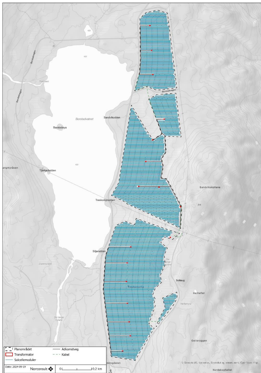
Figur 3-4: Foreløpig layout av Borstad solkraftverk.
