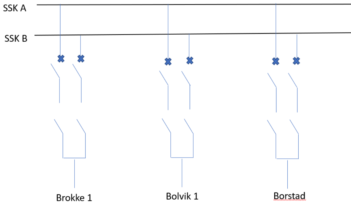
Figur 3-6: Forenklet enlinjeskjema for koblingsstasjon Borstad
