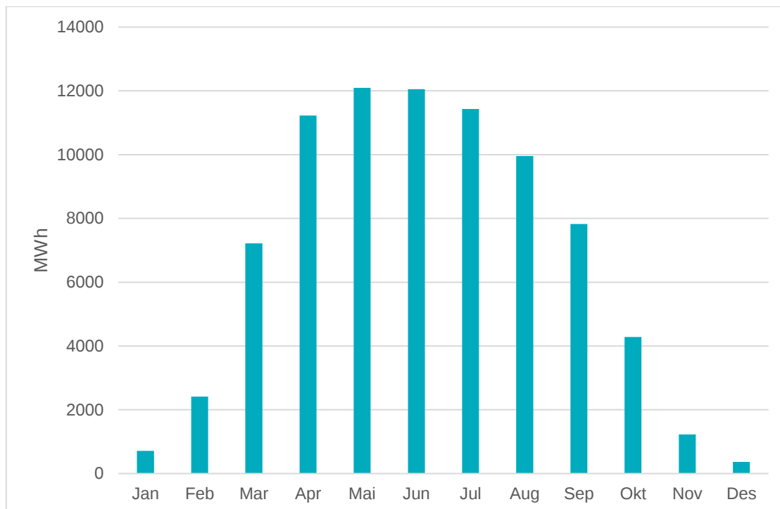
Figur 3-5: Estimert månedlig energiproduksjon
