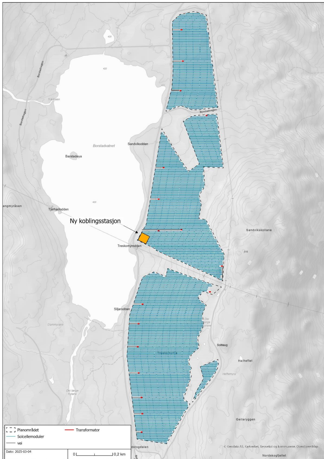
Figur 3-7: Nettilknytning med ny koblingsstasjon som er lokalisert på nordsiden av Brokkeledningene.
