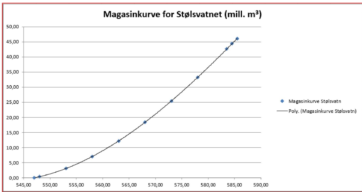
Figur 3 Magasinkurve for Stølsvatnet som er regulert 36,5 meter, mellom kote 547,0 (LRV) og kote 583,5 (HRV). Samla magasinivolum er 42,6 mill.m³
