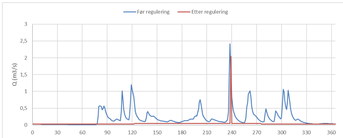
Figur 1 - Vassføringstilhøva nedstraums inntaket til Bøen III i Kaldavatnet før og etter ei regulering i eit tørt år (2010)
