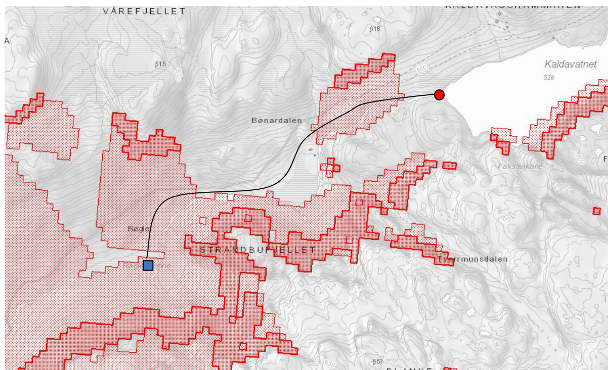
Figur 13 - Aktksomhetsområde for utløpsområde snøskred. Inntak i raudt, nedgrave trase i svart og stasjon markert med blått
