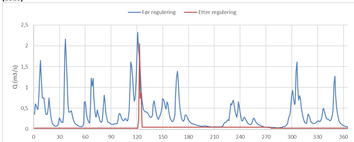
Figur 2 - Vassføringstilhøva nedstraums inntaket til Bøen III i Kaldavatnet før og etter ei regulering i eit normalt år (2000)
