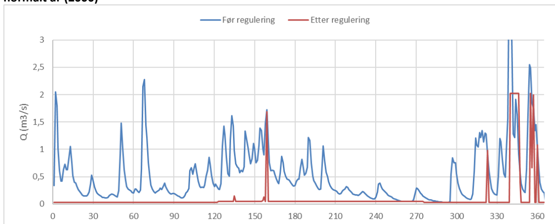
Figur 3 - Vassføringstilhøva nedstraums inntaket til Bøen III i Kaldavatnet før og etter ei utbygging i eit vått år (2015)
