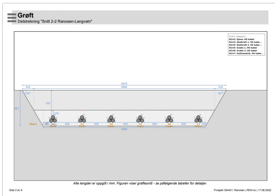
Figur 14: Forlegging av kabelanlegg
