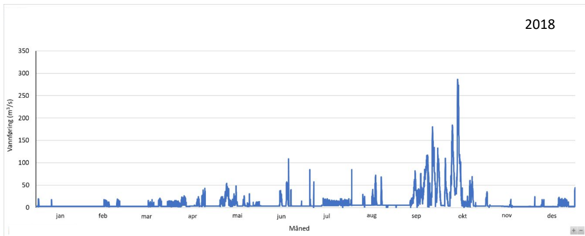
Figur 5. Vannføringsvariasjon i restfeltet målt like oppstrøms Hellandsfossen i 2018. Det er stor unøyaktighet i vannføringer over 5 \text{ m}^3/\text{s} , men grafen viser vannføringsvariasjonen i restfeltet grunnet driften av kraftverket.
