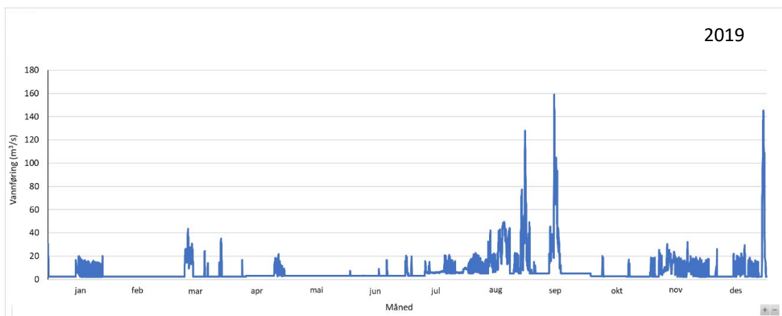
Figur 6. Vannføringsvariasjon i restfeltet målt like oppstrøms Hellandsfossen i 2019. Det er stor unøyaktighet i vannføringer over 5 \text{ m}^3/\text{s} , men grafen viser vannføringsvariasjonen i restfeltet grunnet driften av kraftverket.
