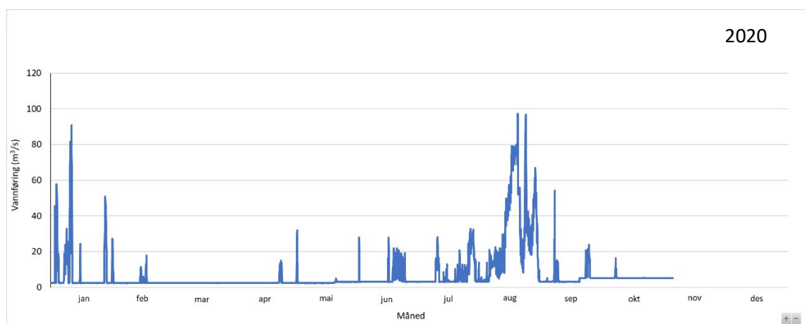
Figur 7. Vannføringsvariasjon i restfeltet målt like oppstrøms Hellandsfossen i 2020. Det er stor unøyaktighet i vannføringer over 5 \text{ m}^3/\text{s} , men grafen viser vannføringsvariasjonen i restfeltet grunnet driften av kraftverket.
