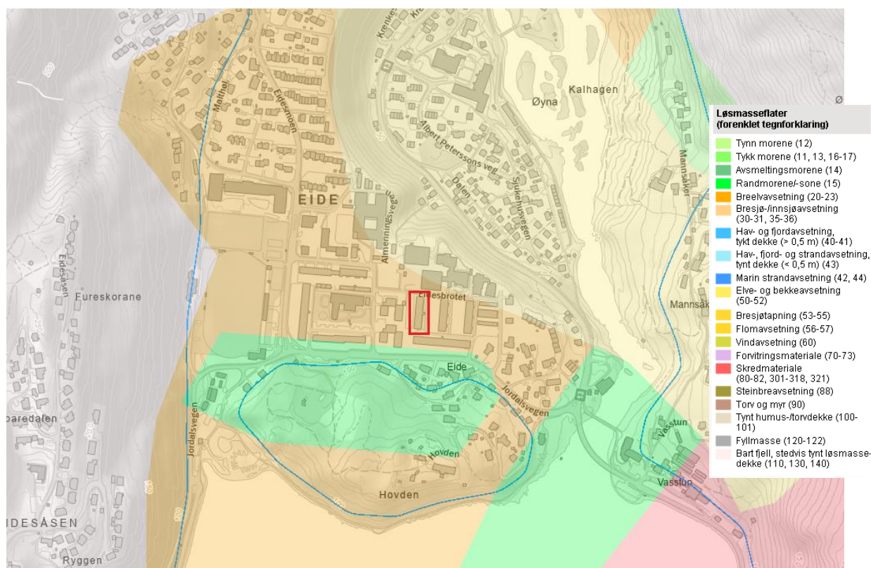
Figur 2: NGUs løsmassekart. Rød sirkel viser tiltakets plassering [2]
