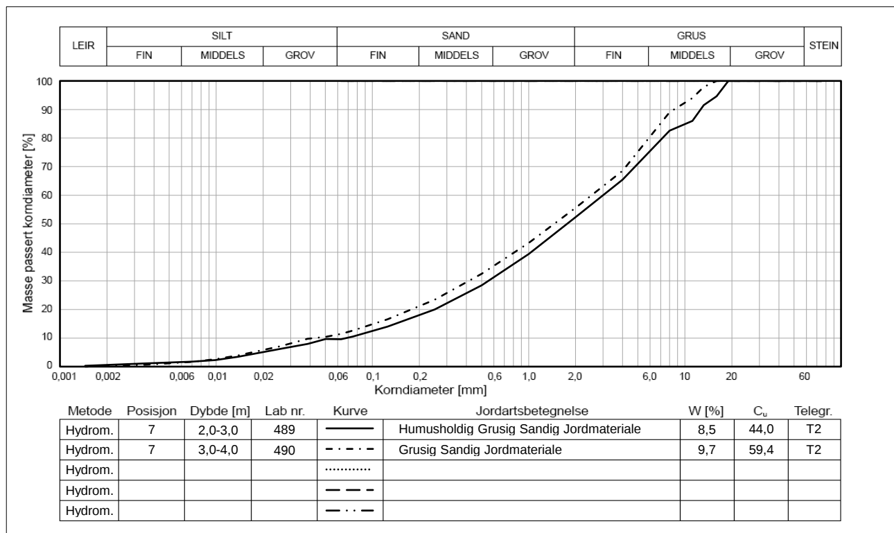
Figur 1 Korngraderingskurver i posisjon 7
