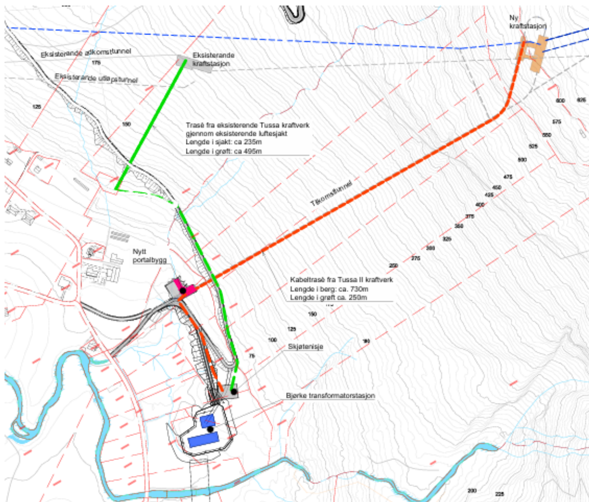
Figur 2: Situasjonsplan for mellombels løysing for tilknytning til nettet på 66 kV. Kilde: Tussa Energi si søknad av 19. februar 2026.
