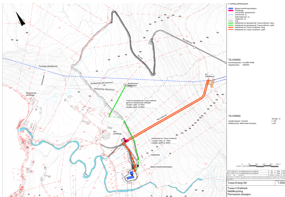
Figur 1: Situasjonsplan som syner omsøkt løysing for ei permanent situasjon med nettknytning. Kilde: Tussa Energi si søknad av 19. februar 2026.
