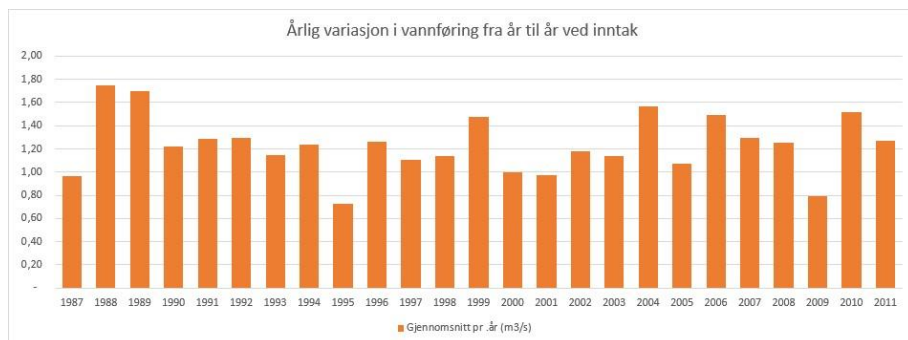
Fig. 5. Årlig variasjon i middelvannføring i Geitelvi. Kilde: Njord vannkraft AS.
