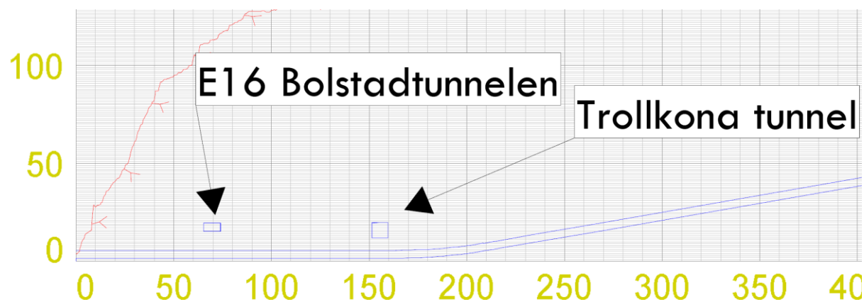
Figur 18. zoomet inn fra P0-P250, fra figur 17. Kryssing under E16 tunnel og under jernbanetunnelen (Trollkona).
