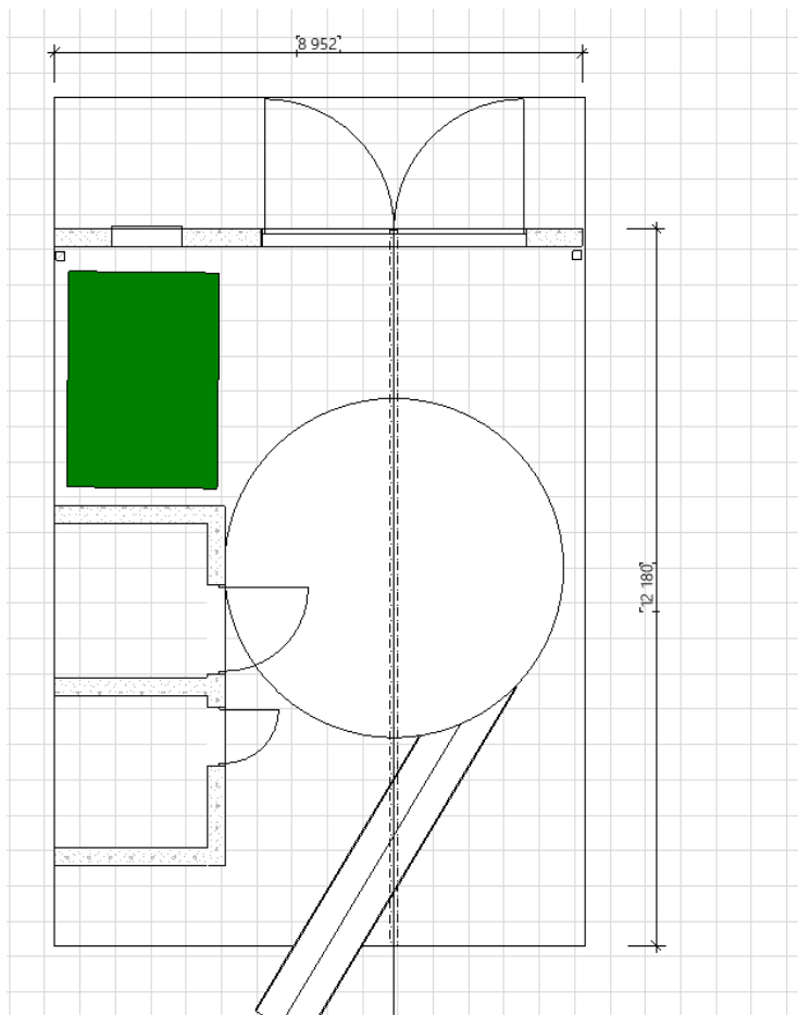
Figur 21 - Foreløpig planskisse av stasjon inne i berg. Port sees øverst, her illustrert med to portblad.
