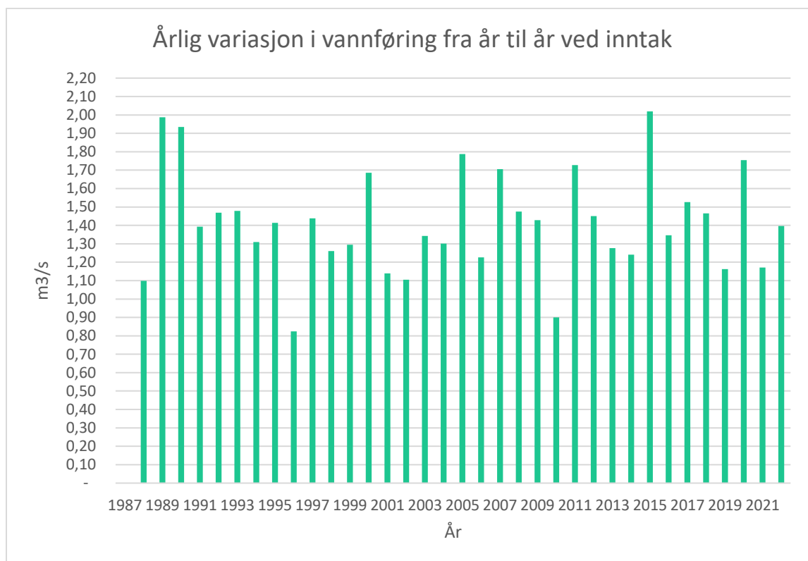
Figur 9: Variasjon i årsmiddelvannføring fra 1988-2021
