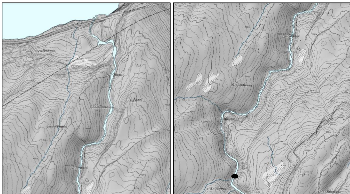
Fig. 20. Topografi og geomorfologi i Geitelvi: nedre avsnitt til venstre, øvre avsnitt til høyre. Inntaket er planlagt like ovenfor Helvetet (vist i kartet til høyre – kote 275). Kilde: Kilden.
