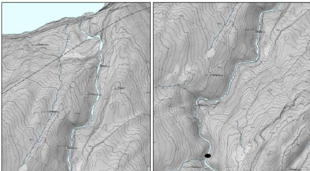
Figur 38 - Topografi og geomorfologi i Geitelvi: nedre del til venstre, øvre avsnitt til høyre. Inntaket markert med sort prikk i figur til høyre. (NNI Resources AS v/A.Håland, 2025) side 26.
