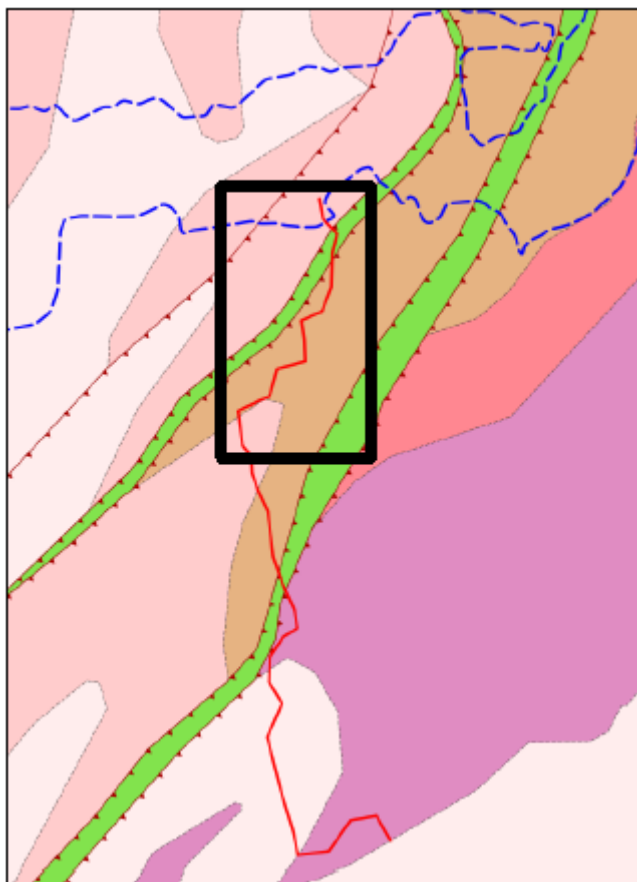
Figur 36 – Berggrunnskart hentet fra NGU.no. Geitelvi tegnet inn som rød strek. Sort avgrenser influensområdet.
