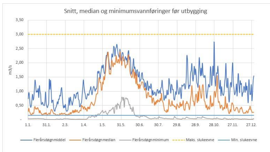
Fig. 7. Flerårsdata vannføring Geitelvi; middel, median og minimum. Planlagt slukeevne lagt inn. Kilde: Njord vannkraft AS.
