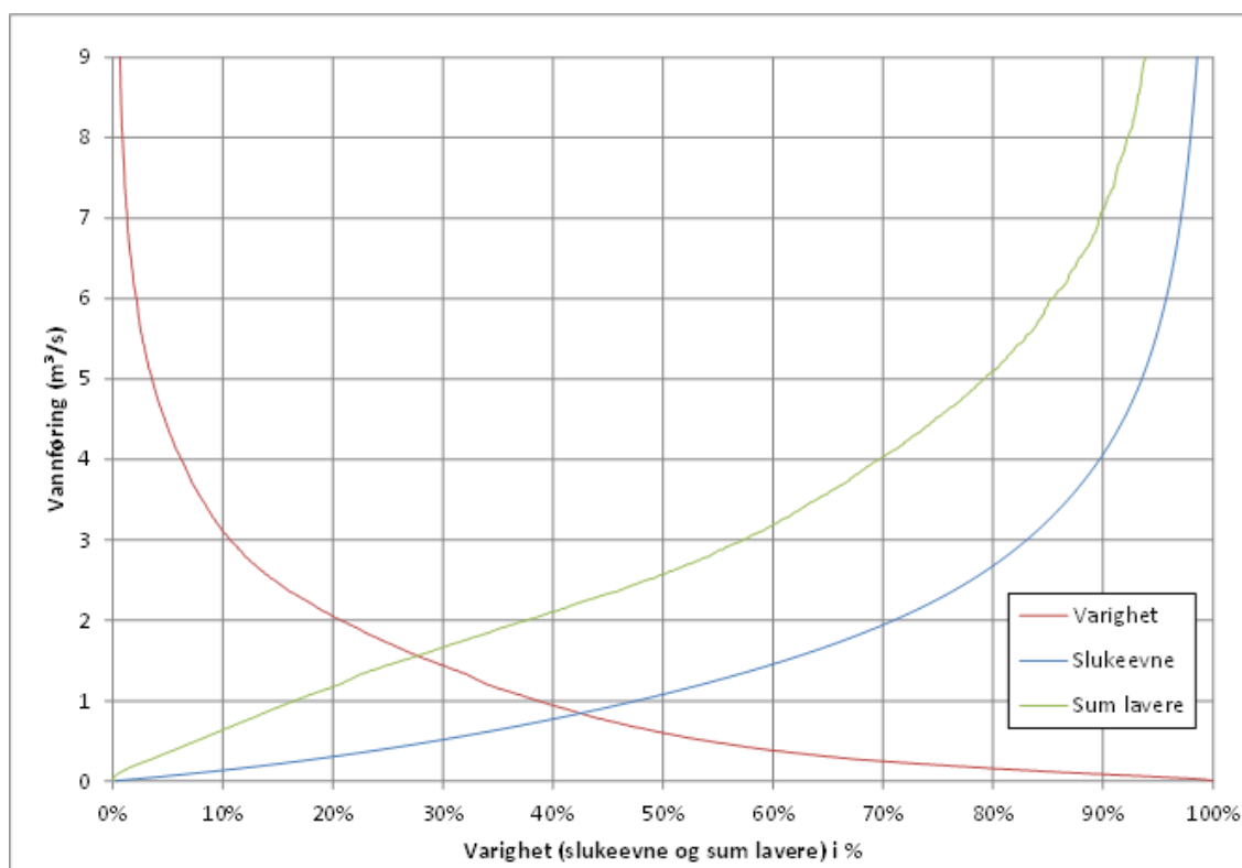
Figur 10: Varighetskurve. (slukeevne og sum lavere i %).
