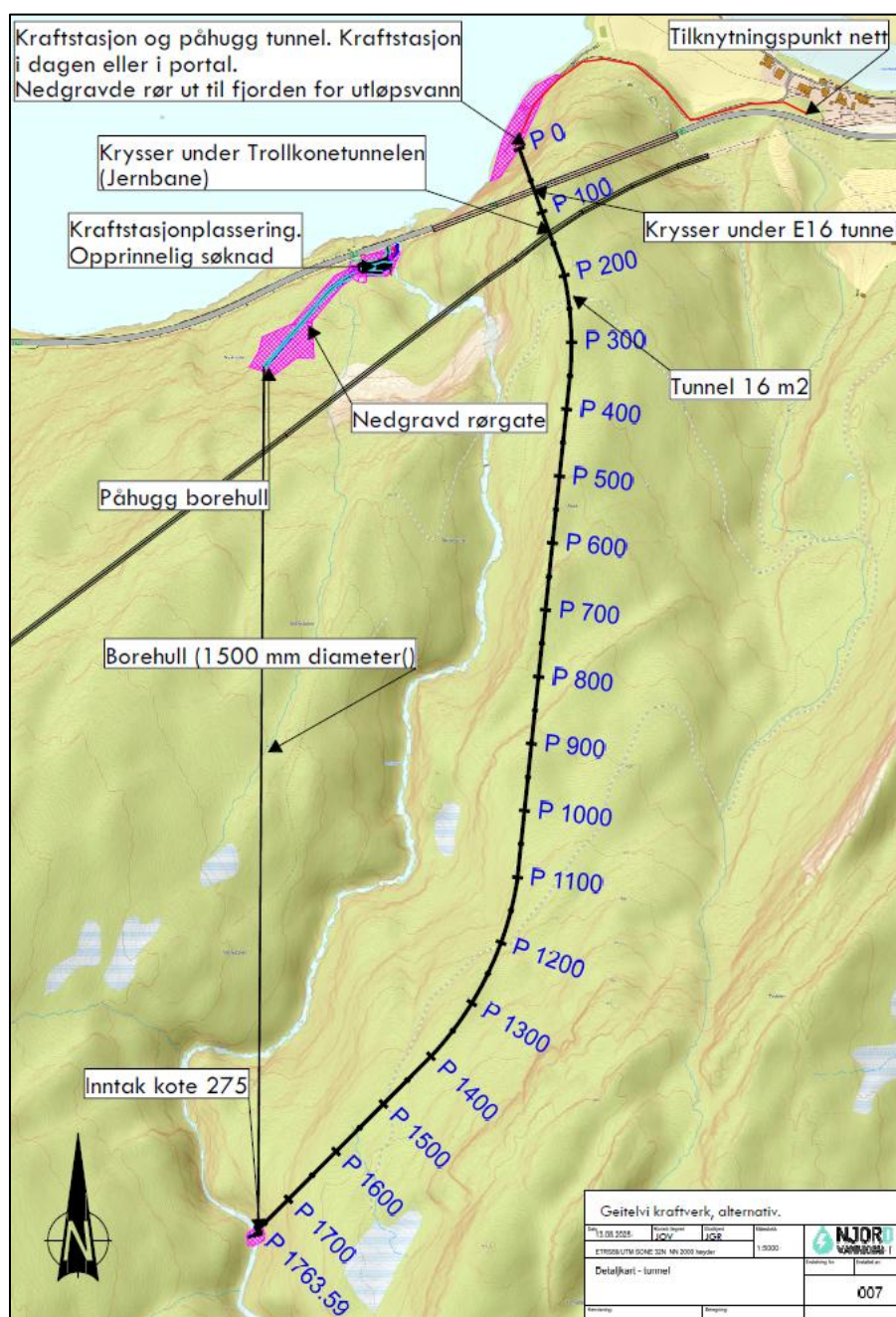
Fig. 8. Opprinnelig plan og nytt alternativ med kraftstasjon ved sjø. Kilde: Njord Vannkraft.
