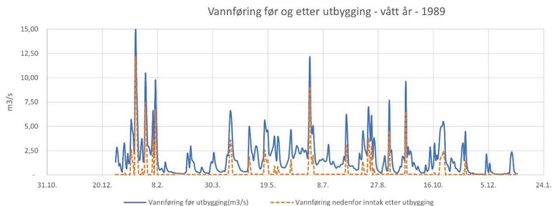
Fig. 11. Vannføring i Geitelvi før og etter utbygging – i et vått år (1989). Kilde: Njord vannkraft AS.
