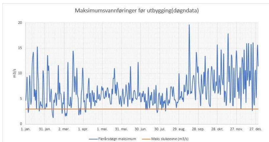
Fig. 6. Maksimum vannføring i Geitelvi gjennom året. Kilde: Njord vannkraft AS.
