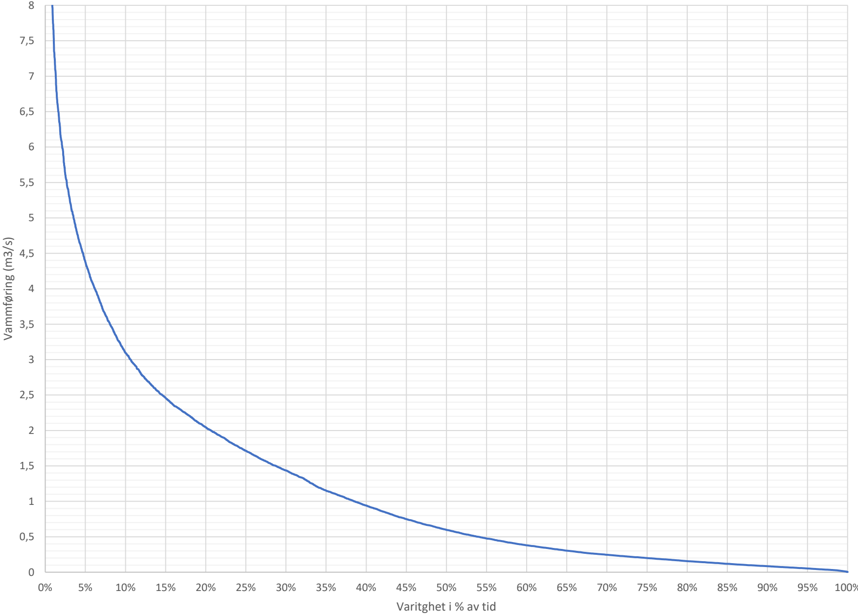
Varighetskurve, Geitelvi ved inntak. (1988-2021)
