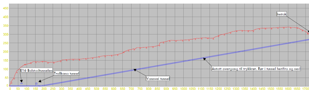
Figur 17 - Lengdeprofil av tunnel. Flat tunnel inn til ca. P180, deretter går tunnel på jevn stigning opp til inntak.
