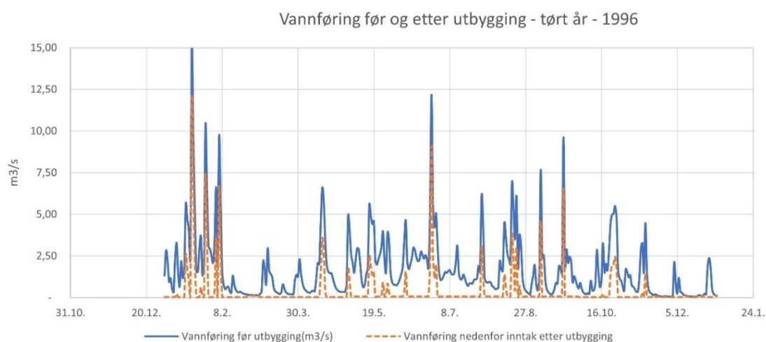
Fig. 13. Vannføring i Geitelvi før og etter utbygging – i et tørt år (1996). Kilde: Njord vannkraft AS
