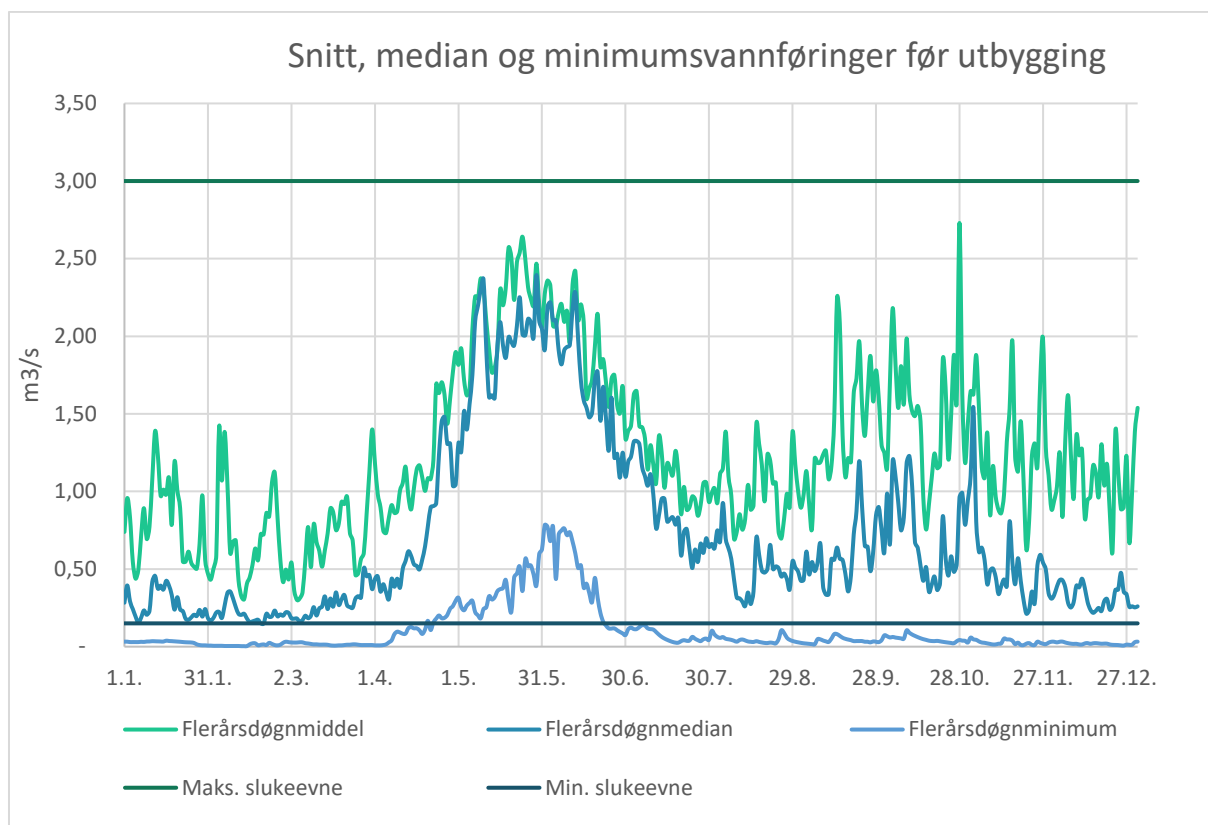
Figur 7: Median og minimumsvannføring samt slukeevne maks 3,0 m 3 /s og min 0,075m 3 /s.
