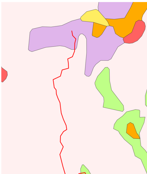
Figur 37 - Løsmasser i landskapet ved Bolstadfjorden og ved Geitelvi. Kilde: (NNI Resources AS v/A.Håland, 2025) s. 26.
