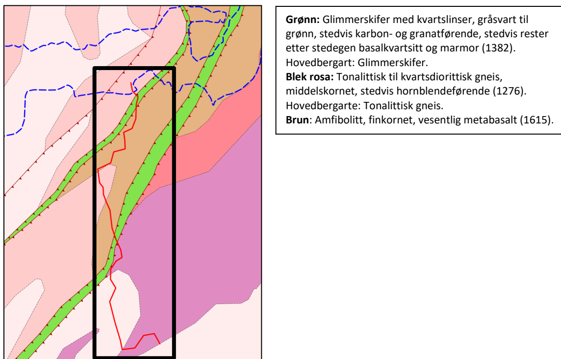
Fig. 18. Berggrunn i landskapet ved Bolstadfjorden, med varierende berggrunn, fra diorittisk og granittisk gneis til noe mer baserik berggrunn som glimmerskifer. Geitelvi er markert med rød linje. Marin grense er også vist. Kartkilde: NGU.
