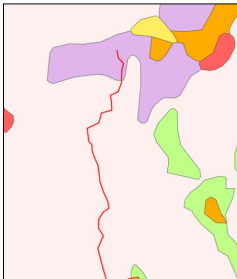
Fig. 19. Løsmasser i landskapet ved Bolstadfjorden og Geitelvi. Kilde: NGU.
