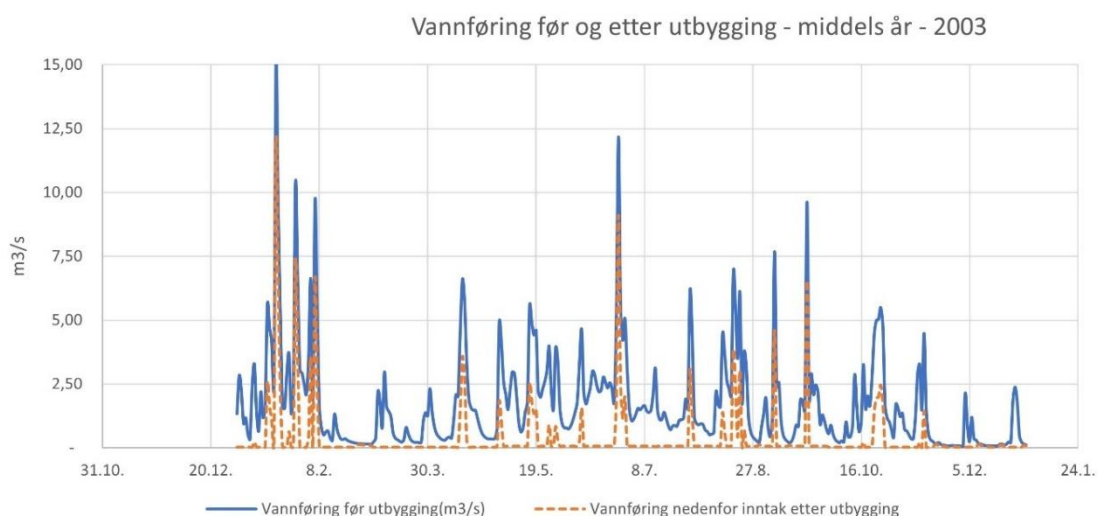
Fig. 12. Vannføring i Geitelvi før og etter utbygging – i et middels nedbørsrikt år (2003). Kilde: Njord vannkraft AS
