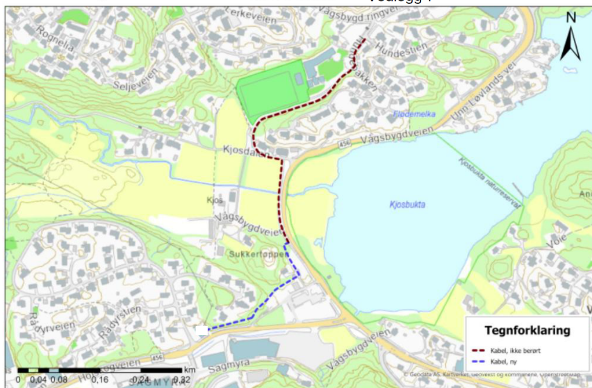
Figur 2. Oversiktskart over hele kabeltraseen etter ombygging, mellom Kjos og Lumber transformatorstasjon. Blå stiplede strek viser omsøkt ledning, rød viser eksisterende ledning. Kilde: Glitre Nett AS sin søknad av 2. juni 2026, vedlegg 1.
