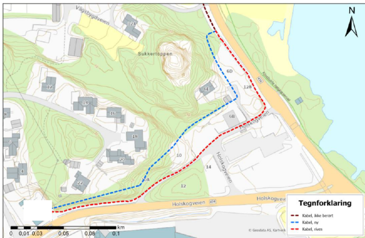
Figur 1. Oversiktskart over konsesjonssøkt tiltak hvor omsøkt jordkabel er markert med blå, stiplet strek, mens eksisterende løsning er markert med rød, stiplet strek. Mørk rød, stiplet strek viser en del av kabelen som skal videreføres. Kilde: Glitre Nett AS sin søknad av 2. juni 2026.
