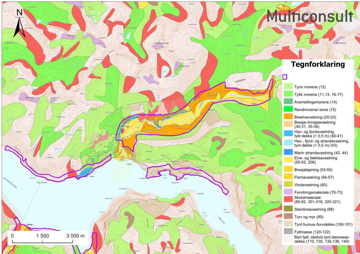
Figur 2. Kvartærgeologisk kartutsnitt over Valldal, Linge og Fjåra [2]
