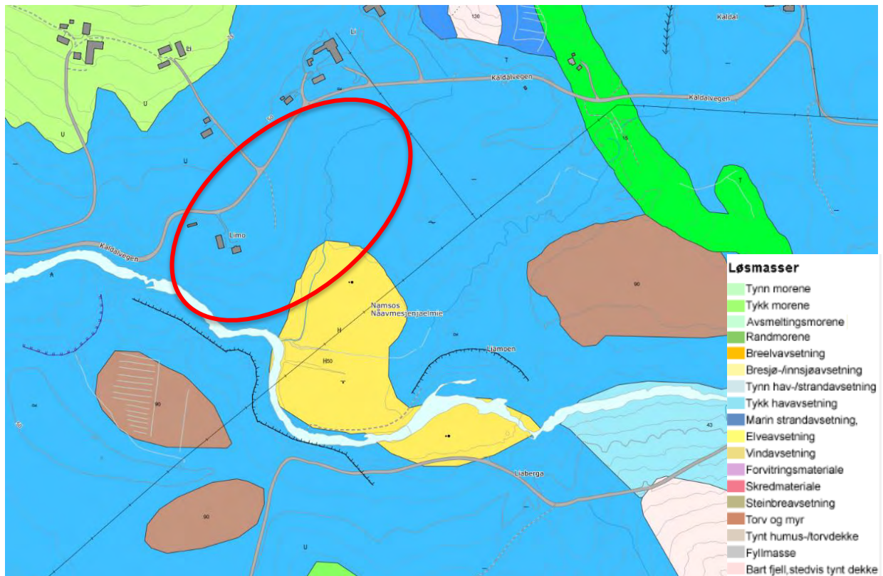
Figur 7-2: Utsnitt av kvartærgeologisk kart – løsmasser. Omtrentlig plassering av kvikkleiresone 1375, er markert med rødt. Kilde: https://geo.ngu.no/kart/
