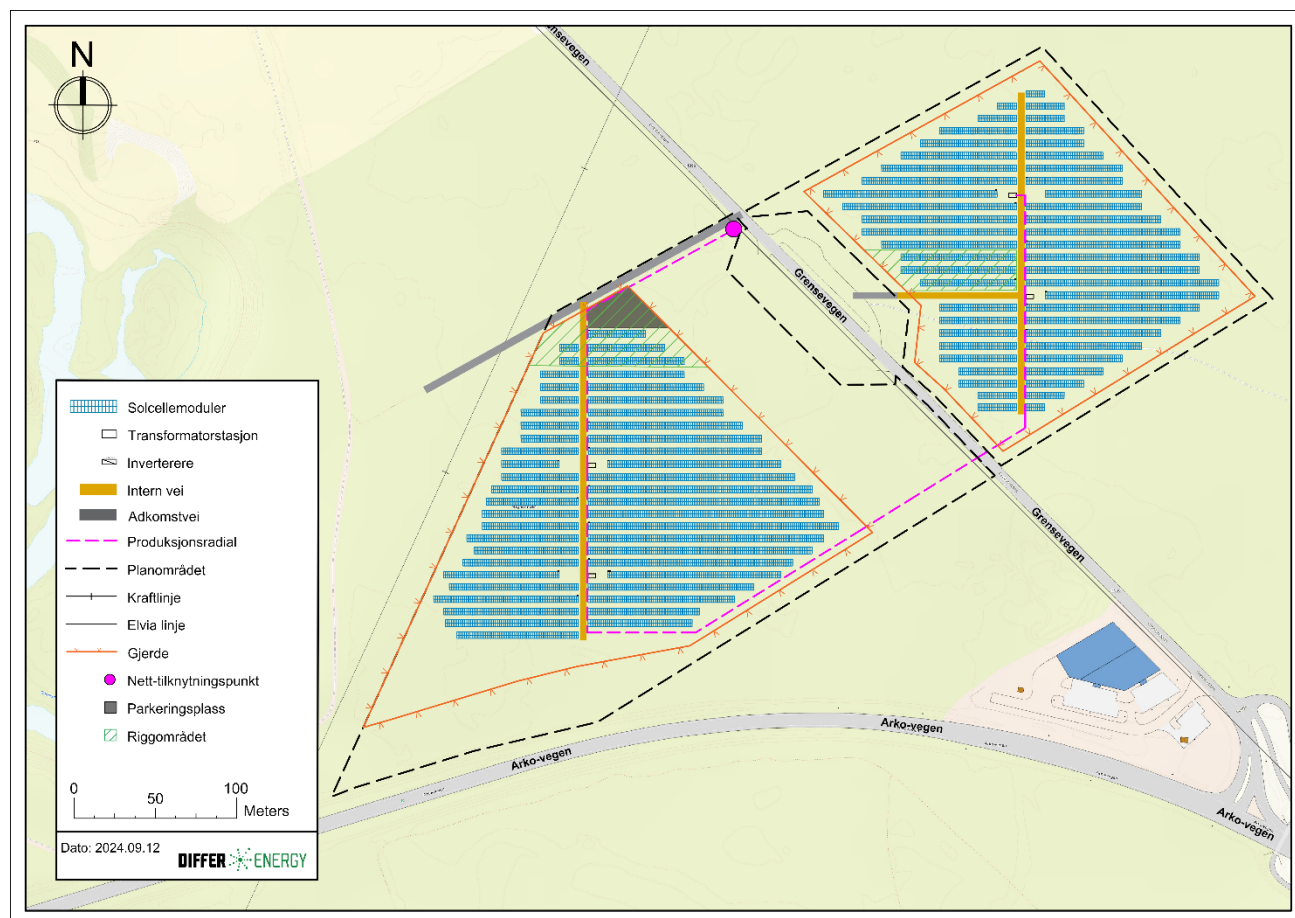
Figur 3. Overordnet oversikt over solkraftverkets installasjon - design
