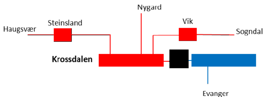
Figur 14: Systemløsning med transmisjonstasjon i Steinsland. Rødt er anleggsdeler på 420 kV, blått er anleggsdeler på 300 kV. Nygard er tilknyttet som produksjonsradial, øvrige anlegg er transmisjonstasjon.
