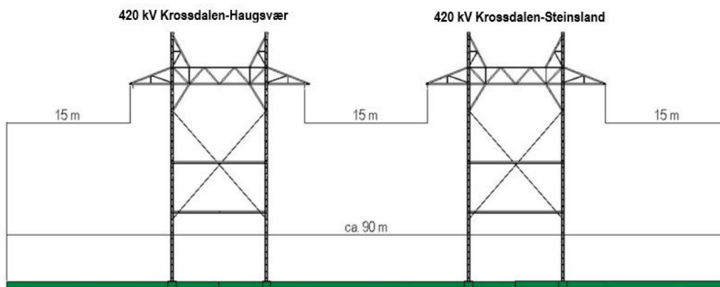
Figur 2: Selvbærende portalmaster
