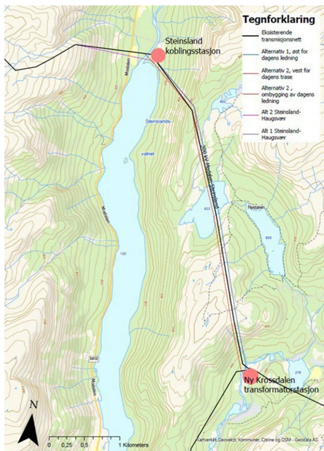
Figur 16: Vurderte ledningsalternativer
