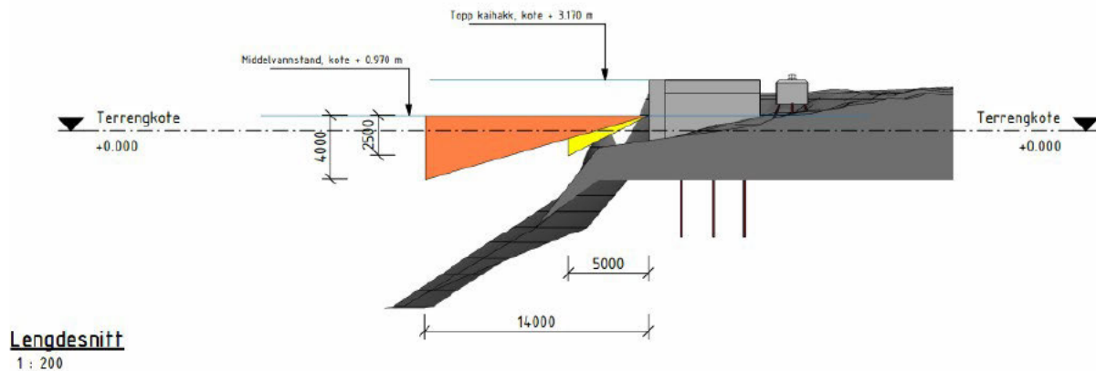
Figur 10: Lengdesnitt av planlagt kaihakk
