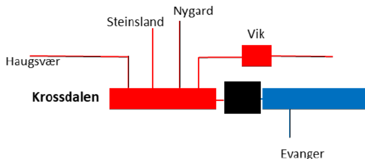
Figur 12: Omsøkt systemløsning. Rødt er anleggsdeler på 420 kV, blått er anleggsdeler på 300 kV. Steinsland og Nygard er tilkoblet som produksjonsanlegg (radialer), øvrige stasjoner er transmisjonsnettstasjoner
