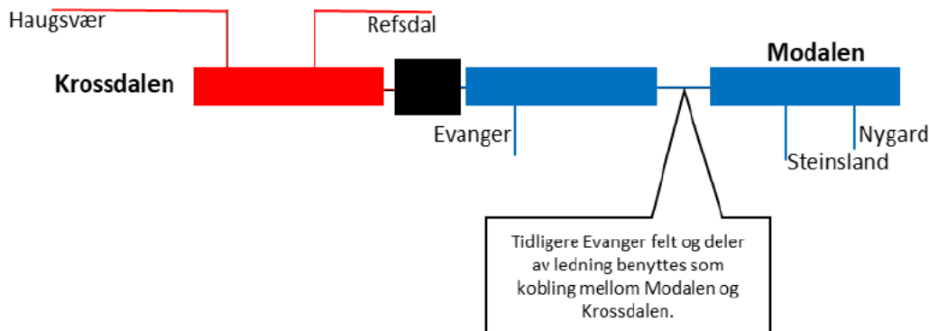
Figur 13: Trinn 1 av trinnvis bygging av Krossdalen stasjon. Rød farge er anlegg med spenning 420 kV, blå farge er anlegg med spenning 300 kV
