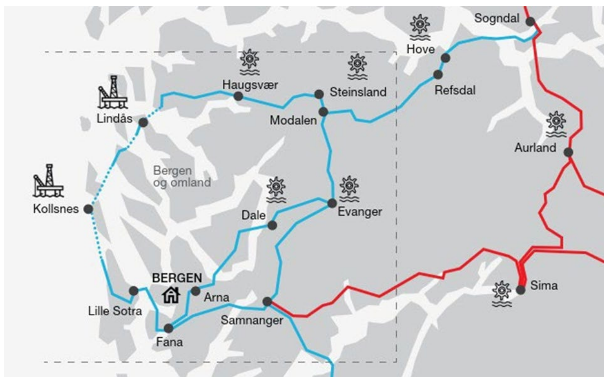
Figur 11: Transmisjonsnett i Bergen og omland, illustrert med blå linje for 300 kV og røde linjer for 420 kV
