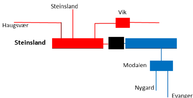
Figur 15: Systemløsning frem til Evanger er på 420 kV hvor transmisjonsnettstasjon blir liggende i Steinsland. Rødt er anleggsdeler på 420 kV, blått er anleggsdeler på 300 kV.
