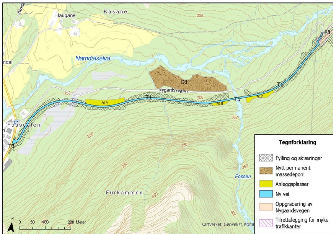
Figur 8: Omsøkt ny del av Nygardsvegen
