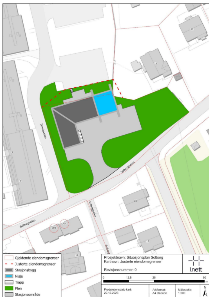
Figur 1: Oversikt over omsøkt plassering av Solborg transformatorstasjon og justering av eiendomsgrenser.
