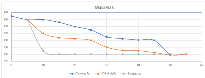
Figur 44: Eksempel på profil for massetak, med opprinnelig terreng, byggegrep og planlagt profil etter istansetting.
