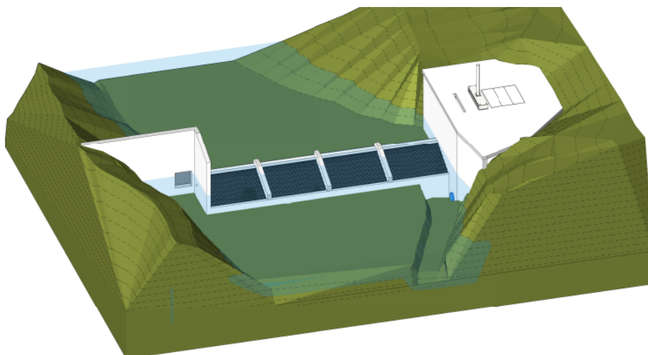
Bilde 3: Skisse av dam i 3D perspektiv sett fra nedside
