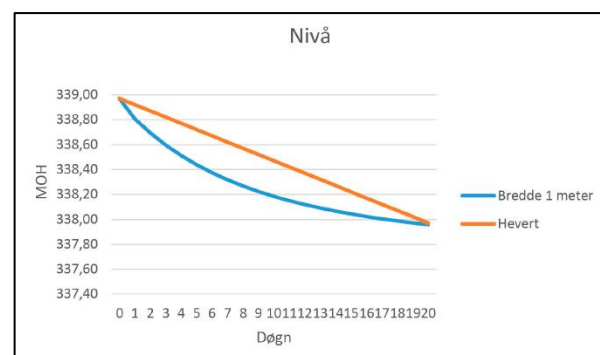
Figur 2: Vannstand i de ytre vannene med hevert og tappeluken.
