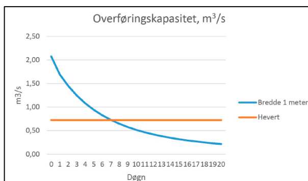
Figur 1: Overføringskapasitet ved hevert og tappeluken.
