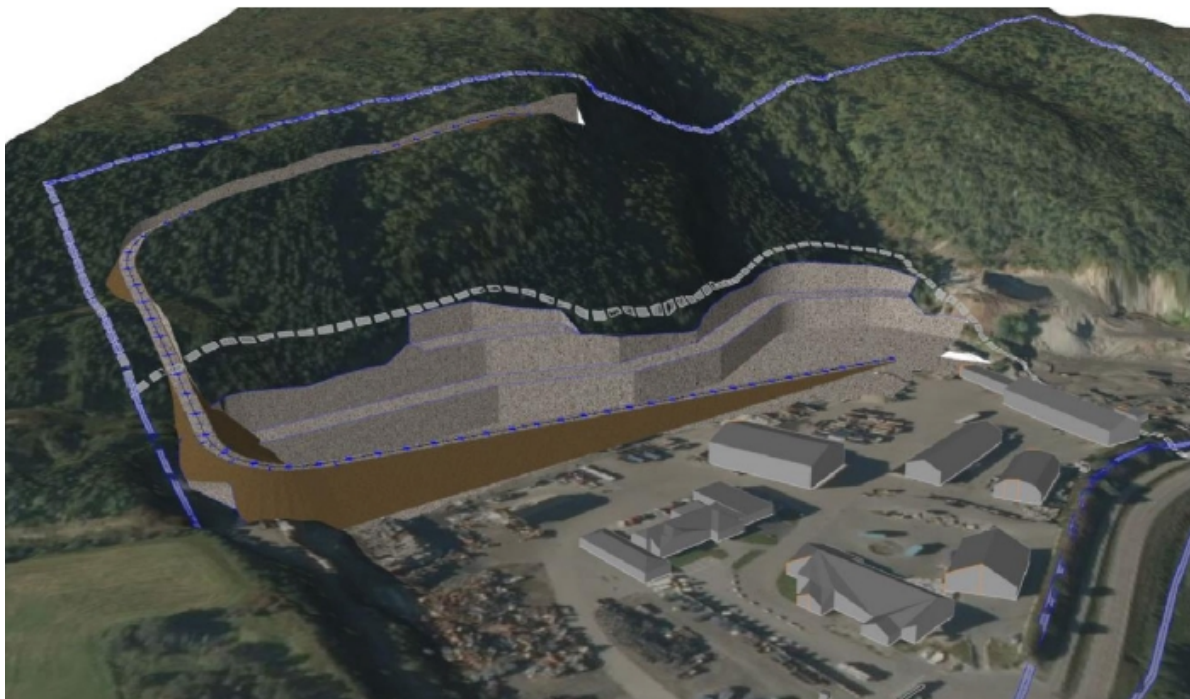
Figur 2: Illustrasjon viser planlagt utbygging av driftsvei for område 3. Parallelsystem slik at den vil bli etablert etter at massene i område 2 er tatt ut.
