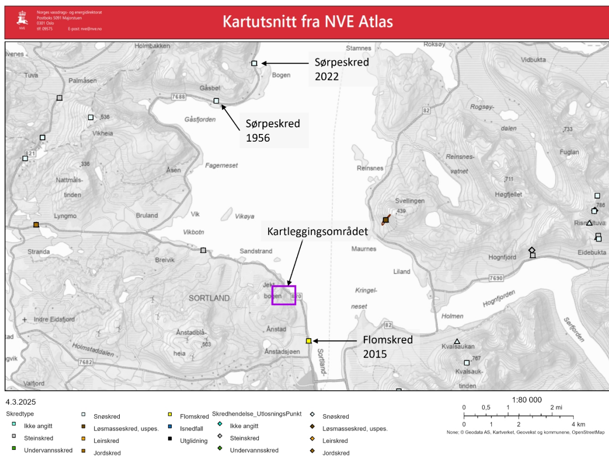
Figur 13: Registrerte skredhendelser i NVE Atlas [3].
