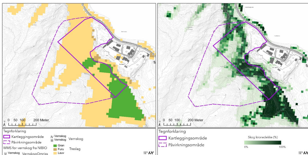
Figur 10: Venstre: skogtype og vernskog. Høyre: kronedekning [10].
