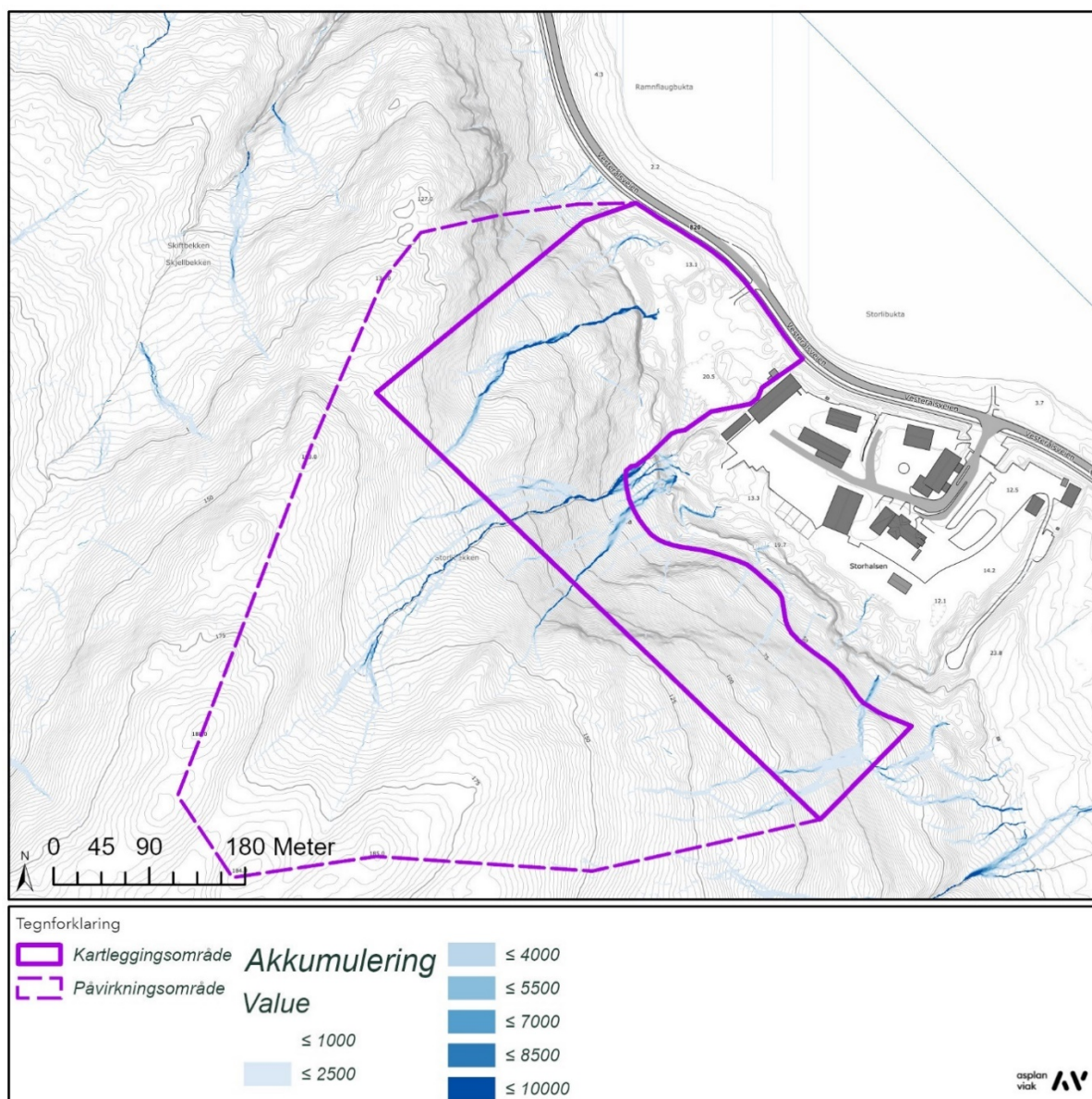
Figur 9: Dreneringsanalyse generert fra terrengmodell i ArcGIS Pro.
