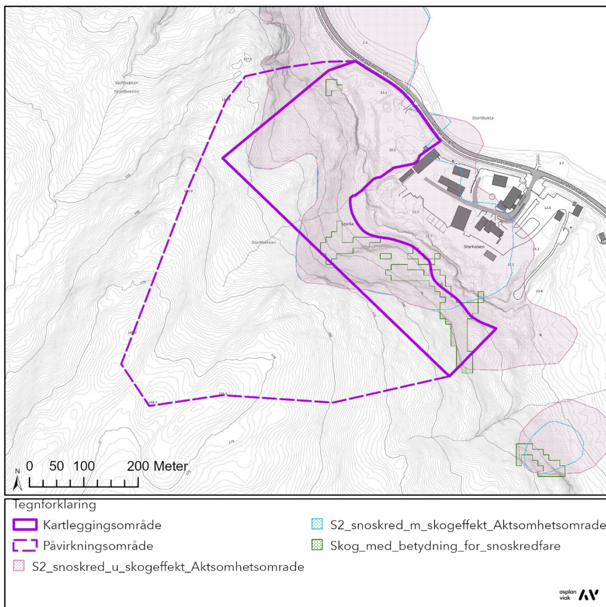
Figur 15: NVEs aktsomhetskart for snøskred (S2 med og uten skog).
