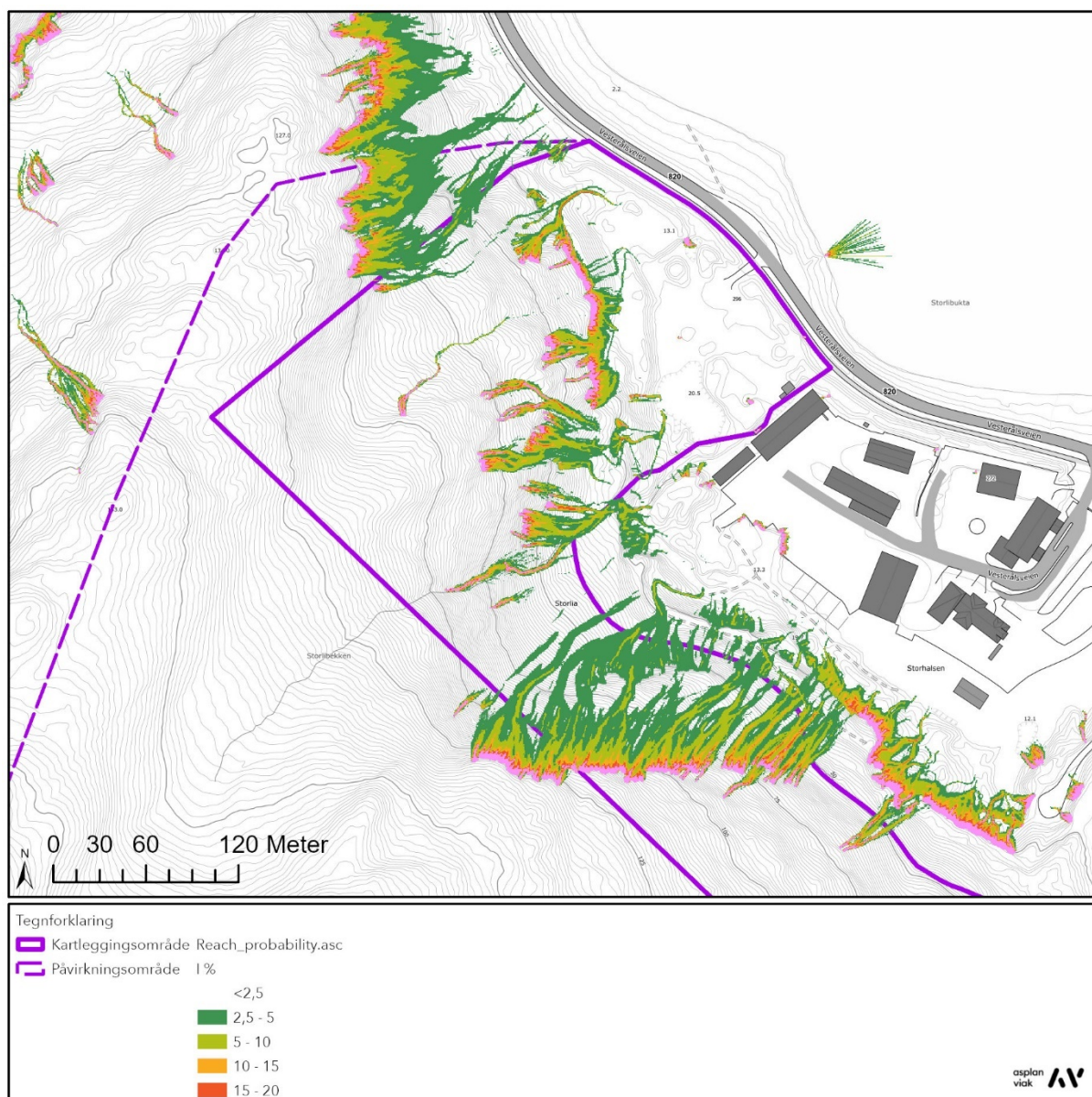
Figur 18: Resultat fra modellering av steinsprang i Rockyfor3D.
