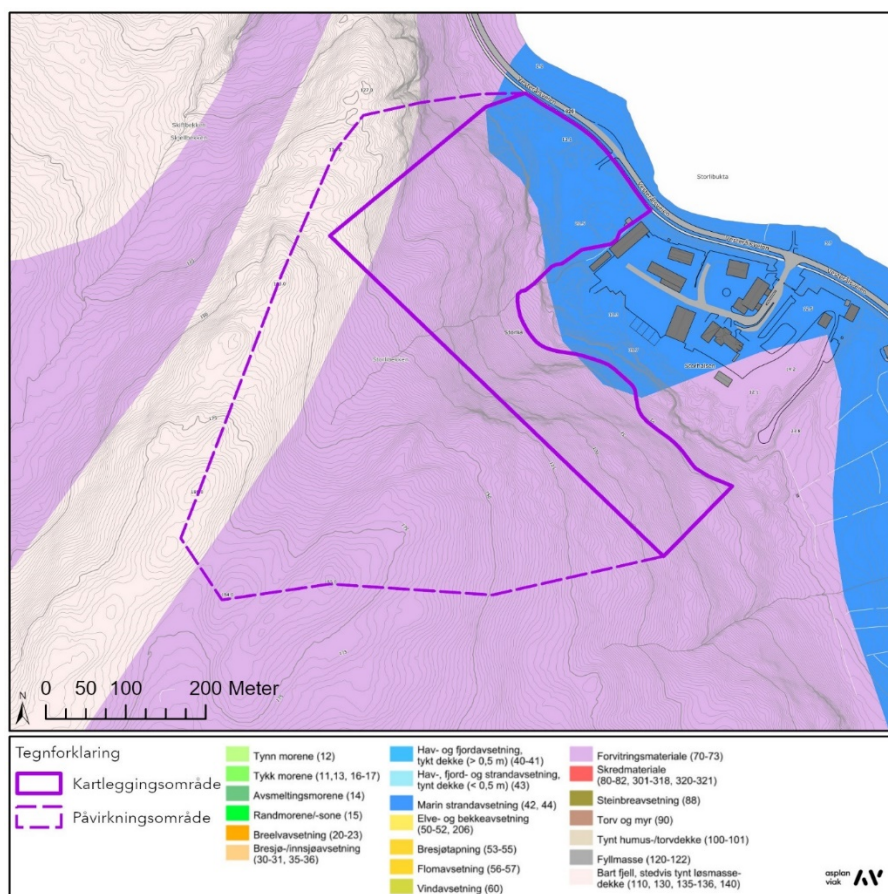
Figur 8: Utsnitt av NGUs løsmassekart (M 1:250 000).
