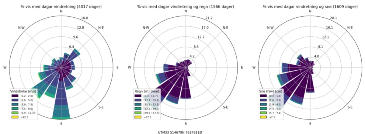
Figur 12: Vindroser. Venstre: generell vindretning. Midtre: vindretning ved regn. Høyre: vindretning ved snø.
