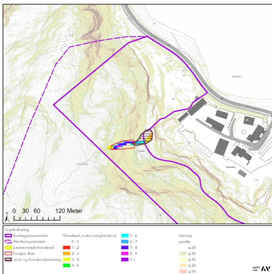
Figur 19: Resultat fra modellering av flomskred i RAMMS::Debris Flow.
