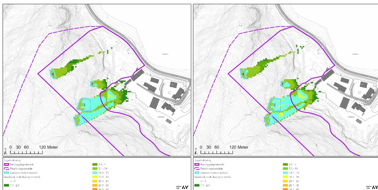
Figur 20: Resultat fra modellering av snøskred i RAMMS Avalanche. Venstre: 100 års scenario. Høyre: 1000 års scenario.
