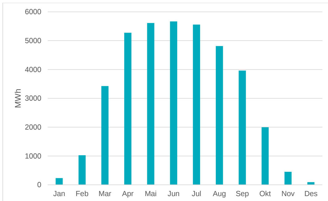
Figur 3-5: Estimert månedlig energiproduksjon
