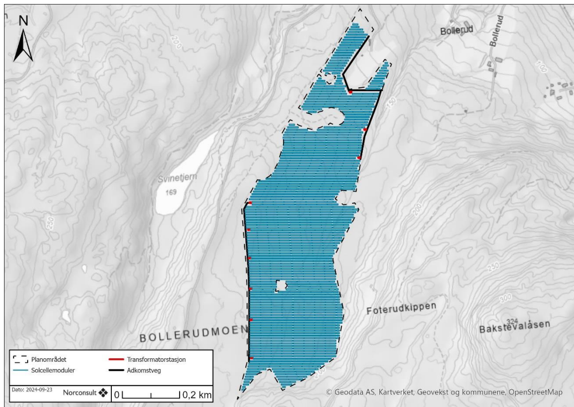
Figur 3-4: Foreløpig layout av Bollerudmoen solkraftverk.
