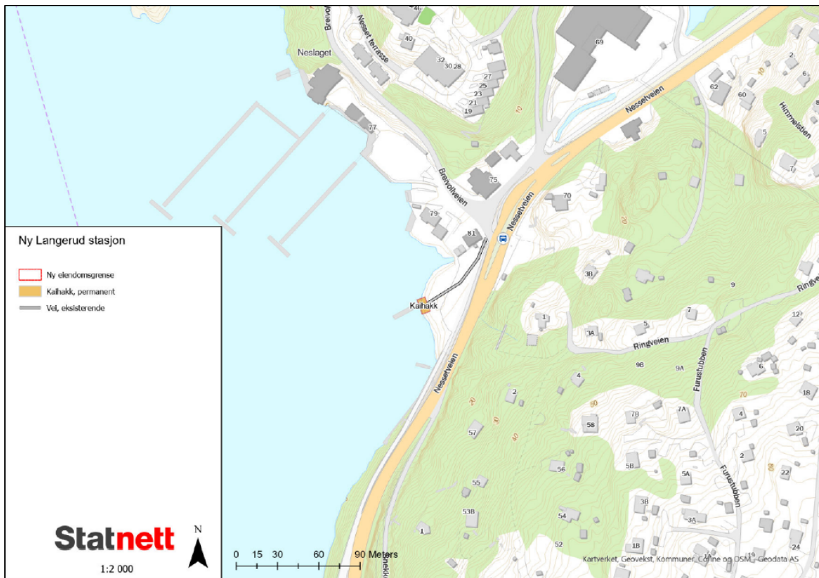
Figur 2: Kartet viser kaihacket som Statnett søker om å bygge ved Nesset i Ås kommune.
