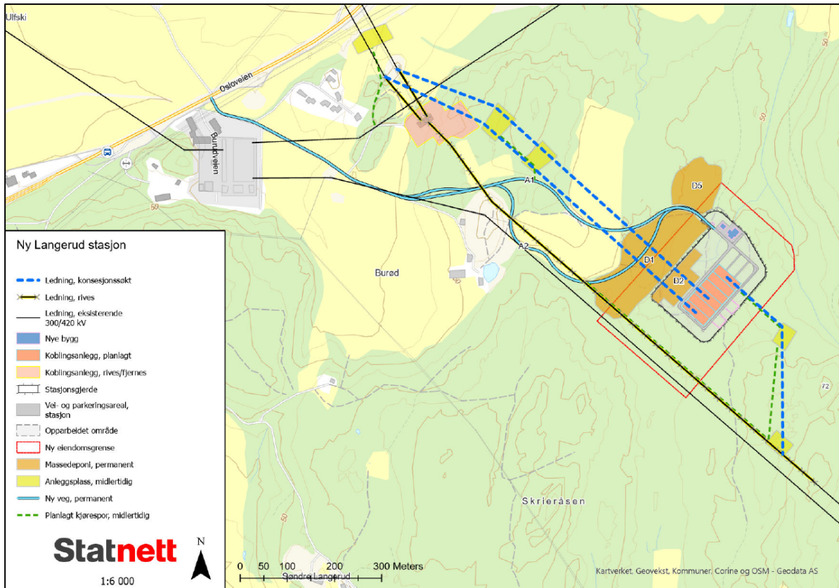
Figur 1: Kartet viser ny Langerud koblingsstasjon i Vestby kommune.
